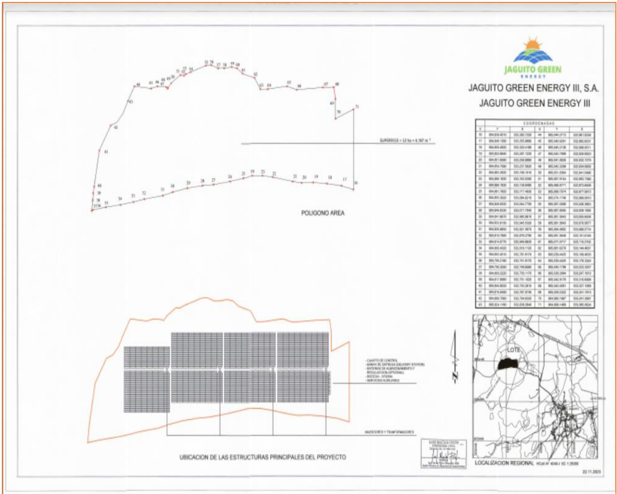
Plano N° 1. Proyecto “PLANTA FOTOVOLTAICA JAGÜTO GREEN ENERGY III”
