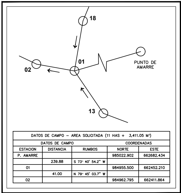
DETALLE DE AMARRE
