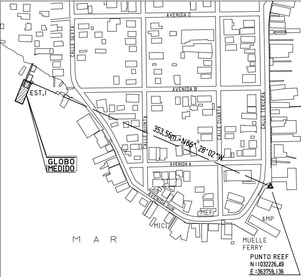
DETALLE DE AMARRE ESCALA: 1 / 3,000
