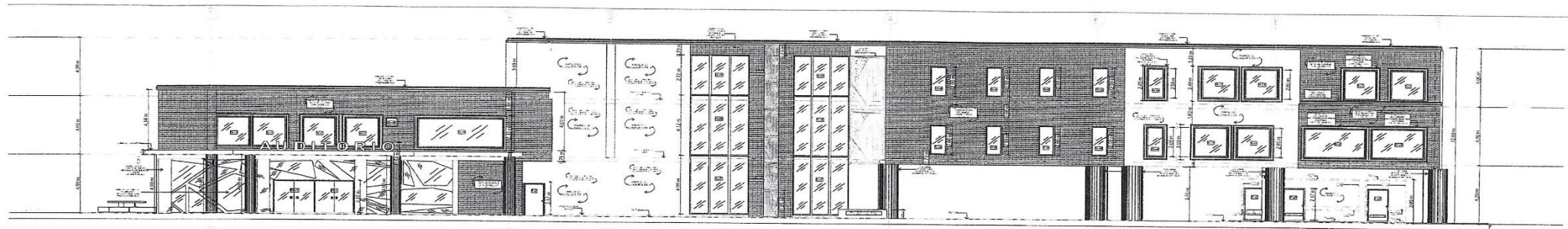
F-01 FACHADA FRONTAL 1:100
