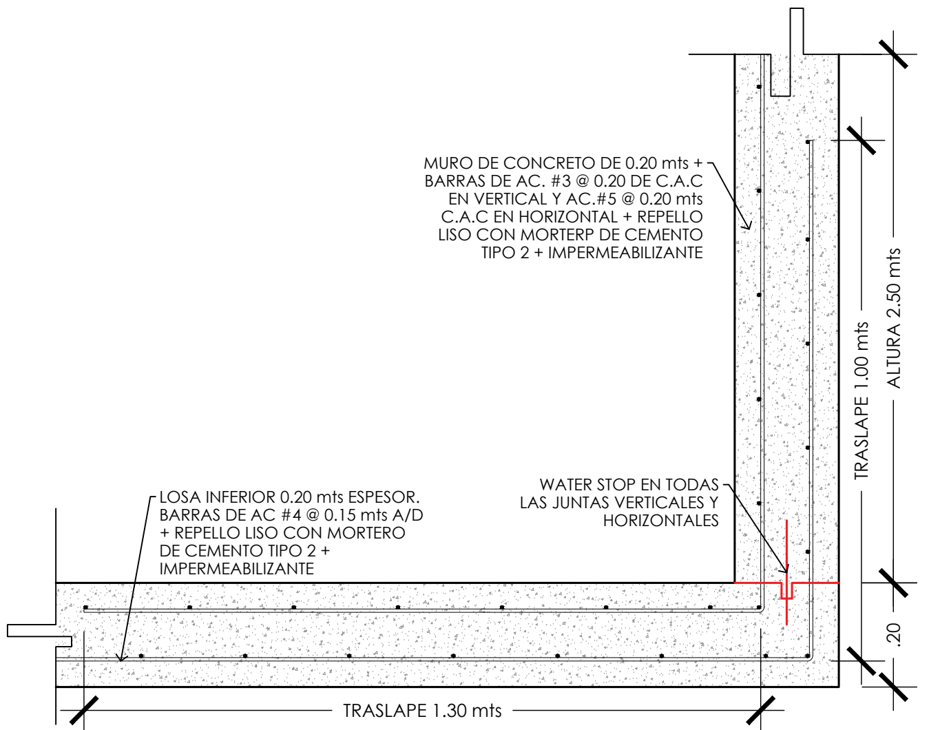
AMPLIACION A (VISTA EN SECCION) ESC: 1/10
