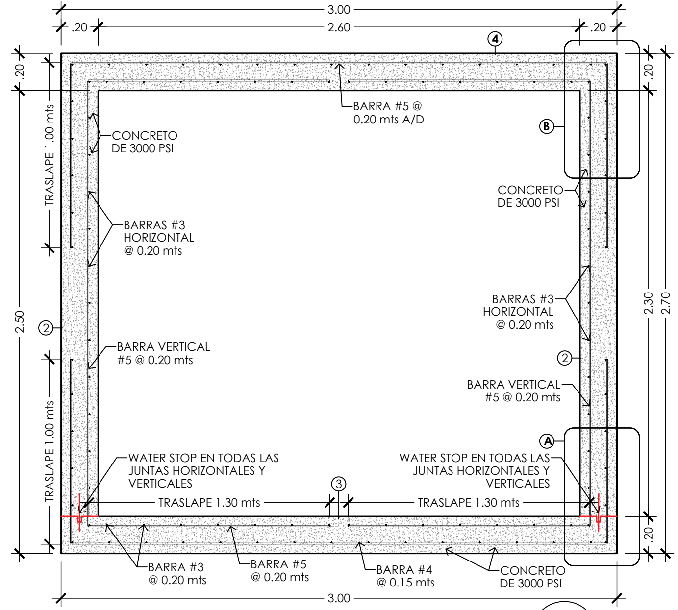
ESQUEMA DE ESTRUCTURA DE FOSA DM 01 ESC: 1/25
