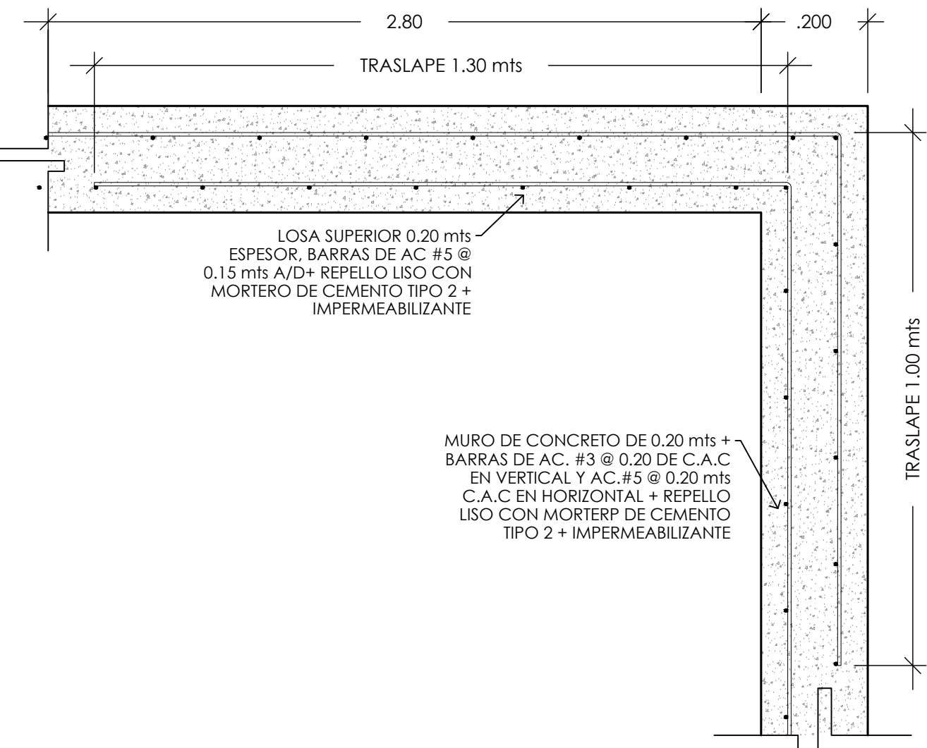
AMPLIACION B (VISTA EN SECCION) ESC: 1/10
