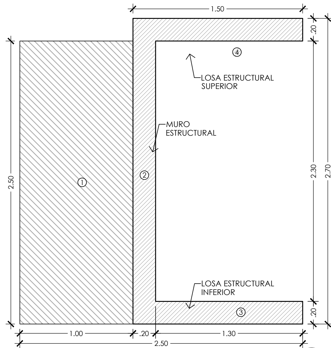
ESQUEMA DE ESTRUCTURA DE LOSA DM 01 ESC: 1/20
