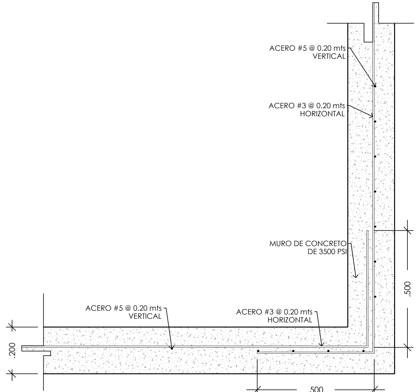
DETALLE VISTA EN PLANTA ESC: 1/10
