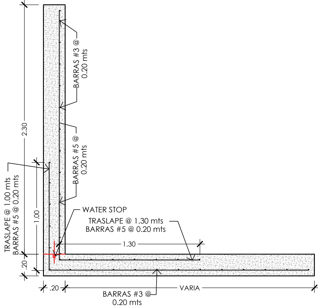
ESQUEMA DE ESTRUCTURA DE FOSA
