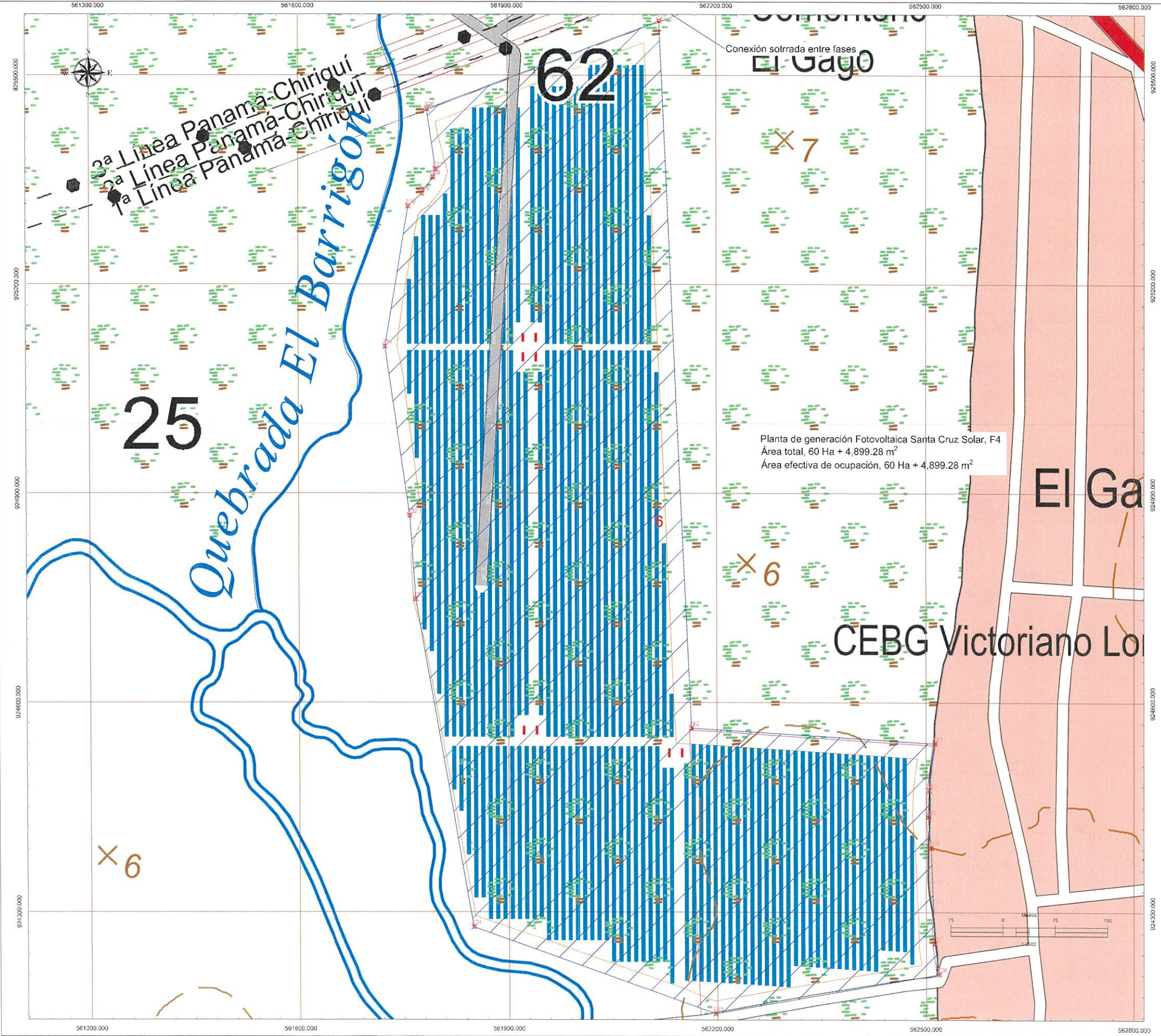
"PLANTA DE GENERACION FOTOVOLTAICA, SANTA CRUZ SOLAR" F4
