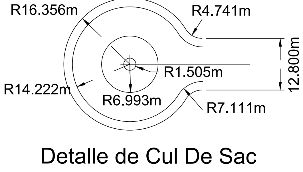
Detalle de Cul De Sac
