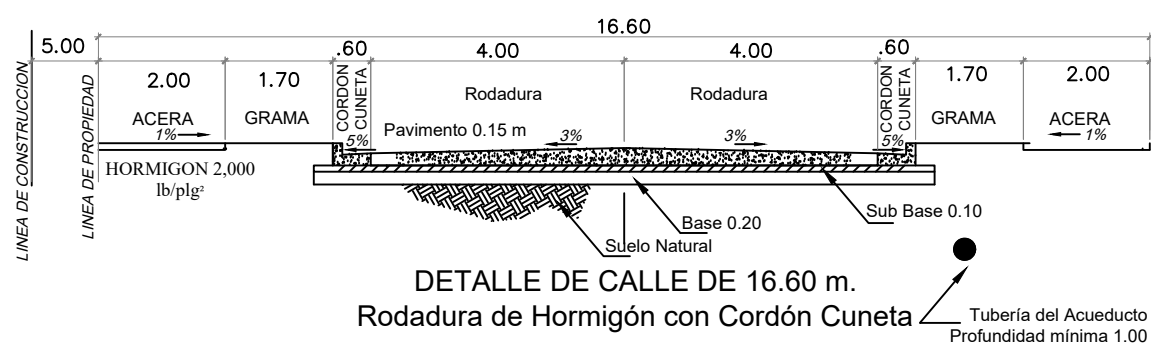
Detalle de Calle de 16.60 m. Rodadura de Hormigón con Cordon Cuneta
