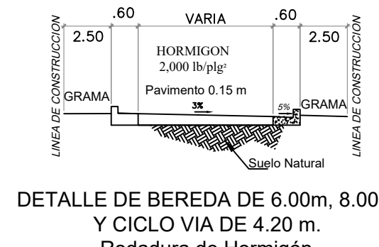
Detalle de Bereda de 6.00m, 8.00m Y CICLO DE VÍA DE 4.20 m. Rodadura de Hormigón
