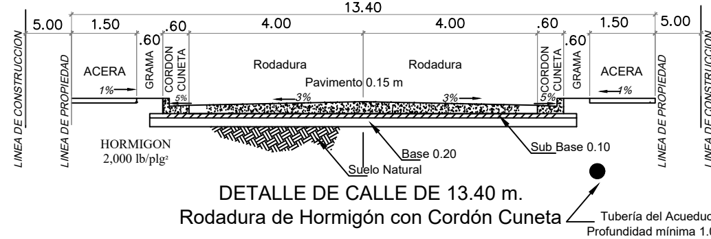
Detalle de Calle de 13.40 m. Rodadura de Hormigón con Cordon Cuneta
