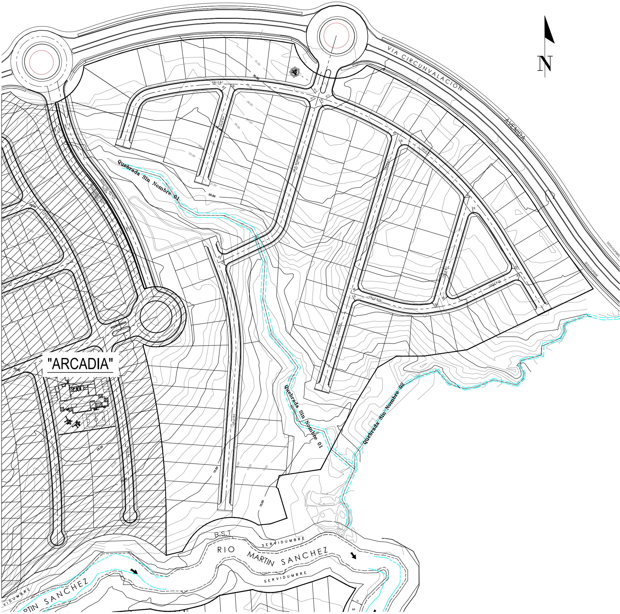
LOTIFICACION GENERAL ESCALA 1:2000
