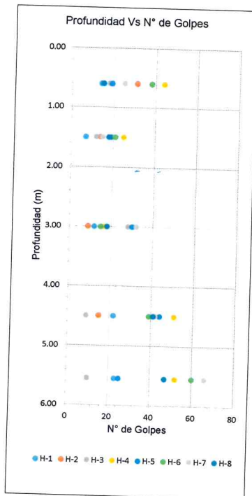
Gráfica N°1: Profundidad Vs N° de Golpes
