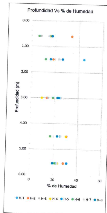
Gráfica N°2: Profundidad Vs % de Humedad
