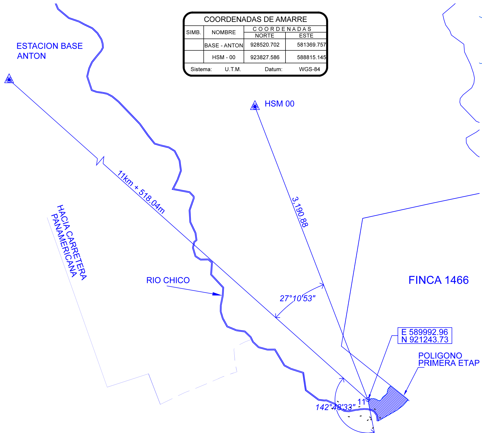
DETALLE DE AMARRE ESCALA= 1:20,000
