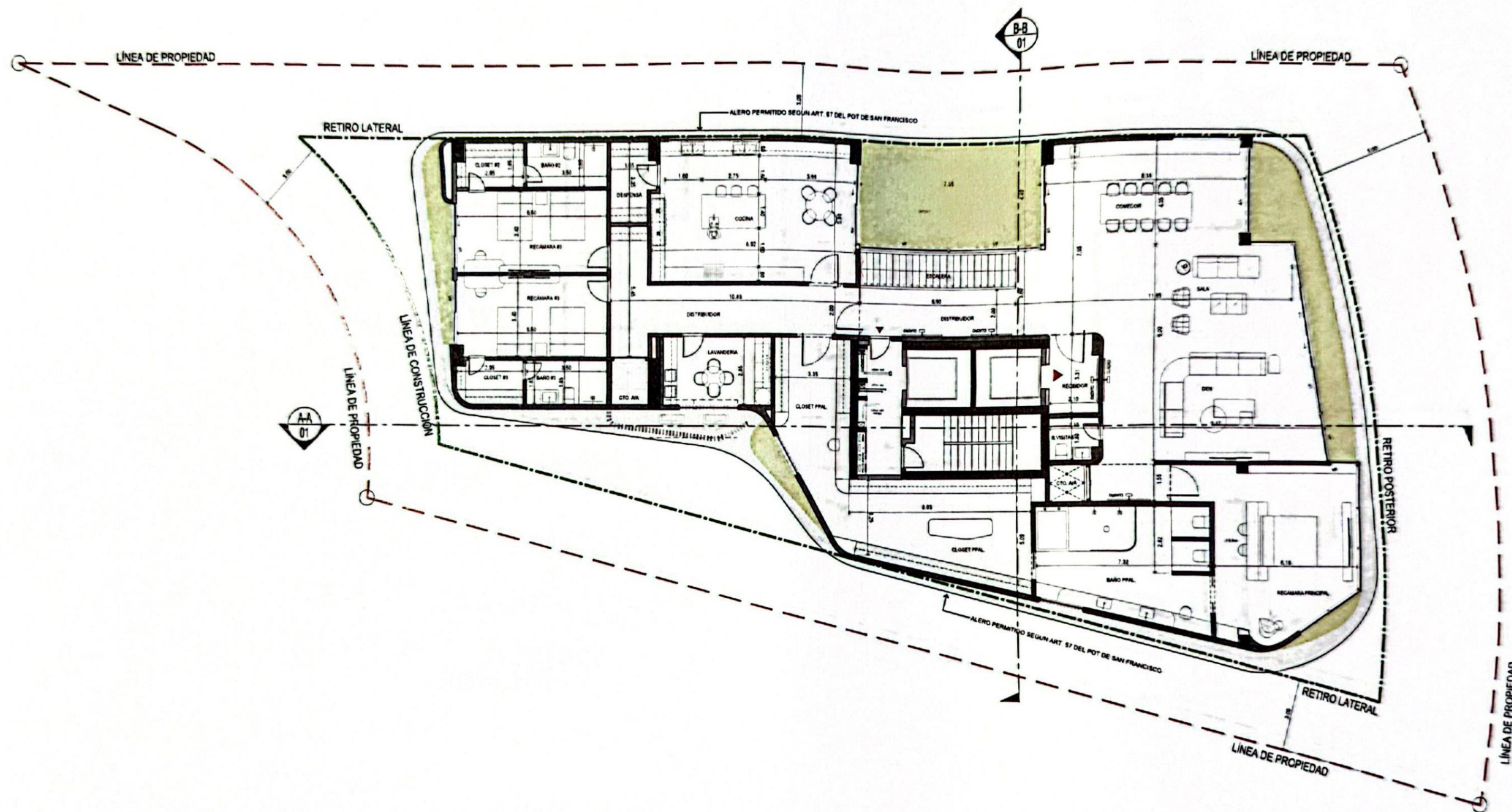
PLANTA ARQUITECTÓNICA N500 ESC. 1/75
