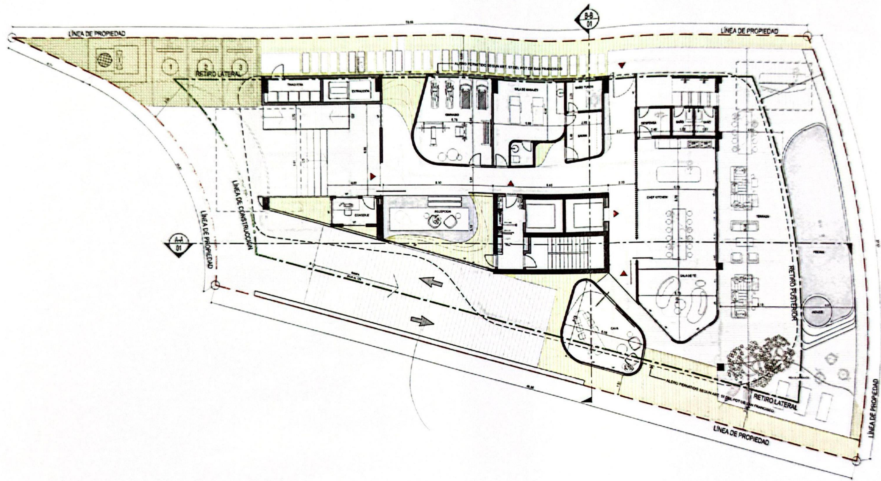
PLANTA ARQUITECTÓNICA N000 ESC: 1/75
