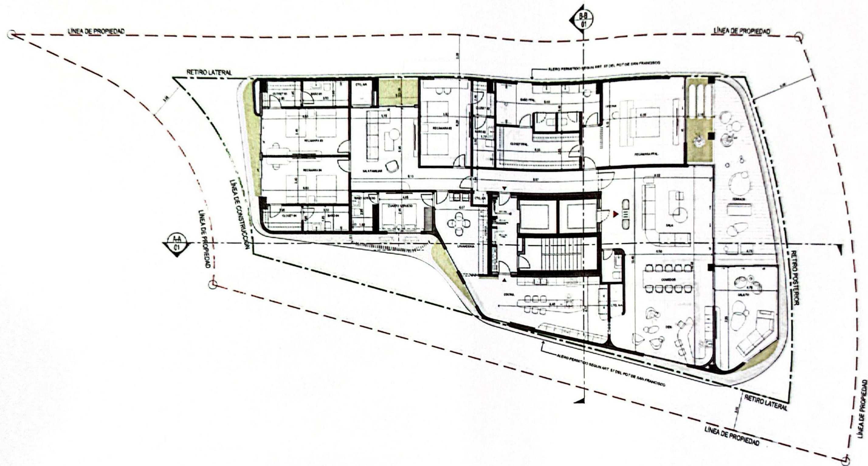
PLANTA ARQUITECTÓNICA N100-400 ESC 1/75
