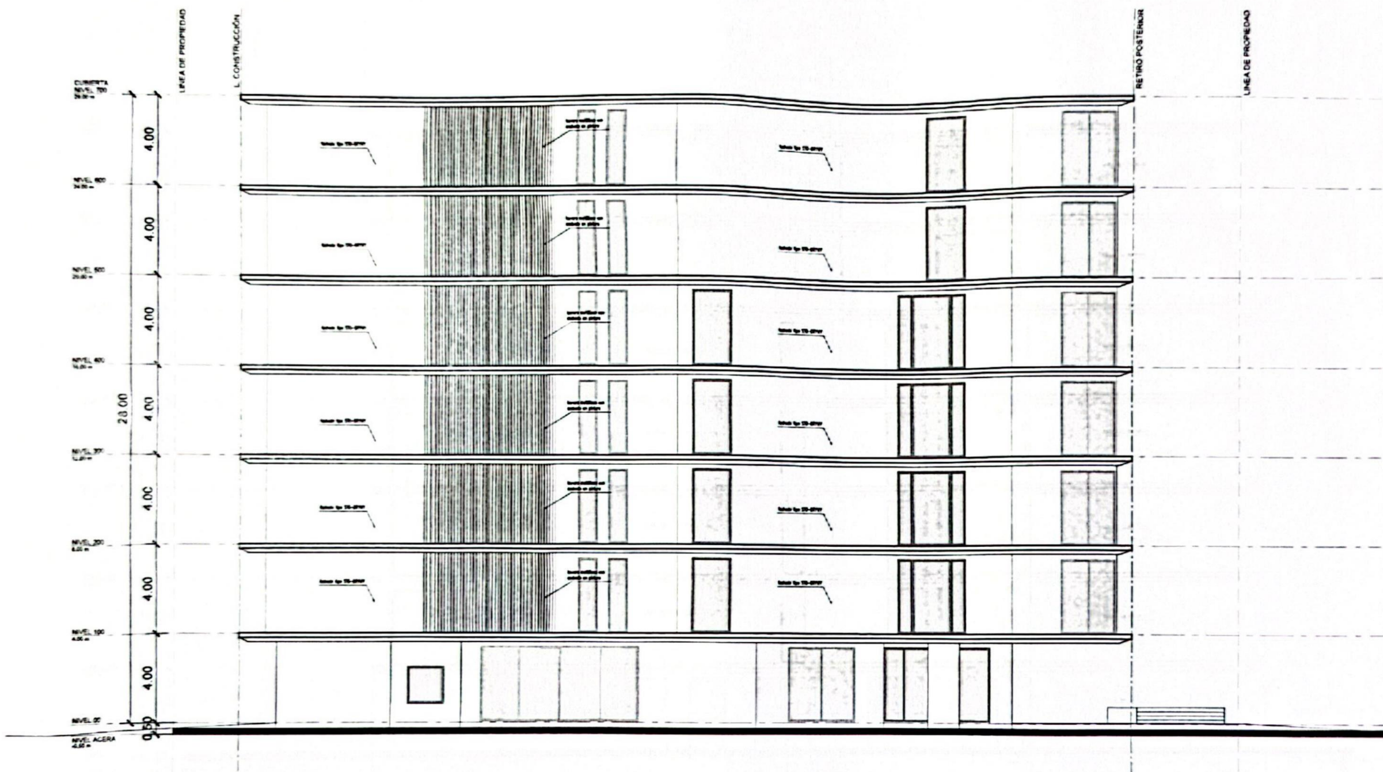
ELEVACIÓN LATERAL DERECHA ESC 1/75
