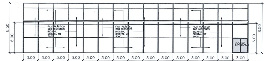
ELEVACION LATERAL DERECHA MODULO I ESC. 1:200
