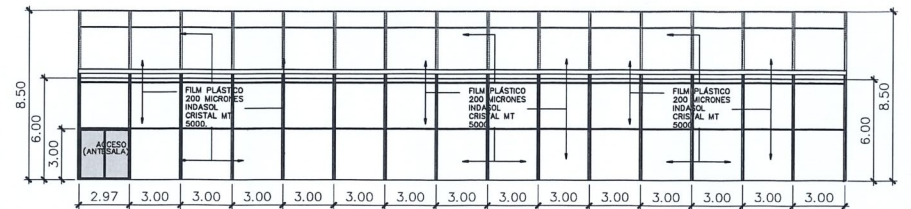
ELEVACION LATERAL IZQUIERDA MODULO I ESC. 1:200
