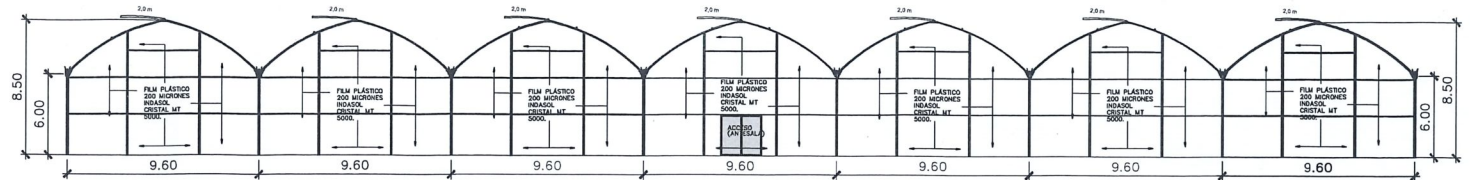
ELEVACION FRONTAL MODULO II
