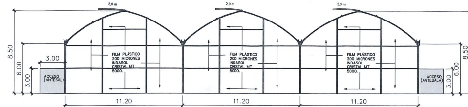
ELEVACION FRONTAL MODULO I ESC. 1:200
