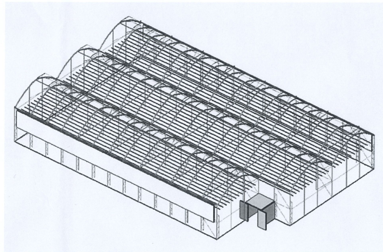
ISOMETRICO DEL MODULO I ESC. 1:200
