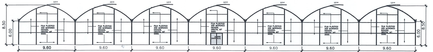
ELEVACION POSTERIOR MODULO II
