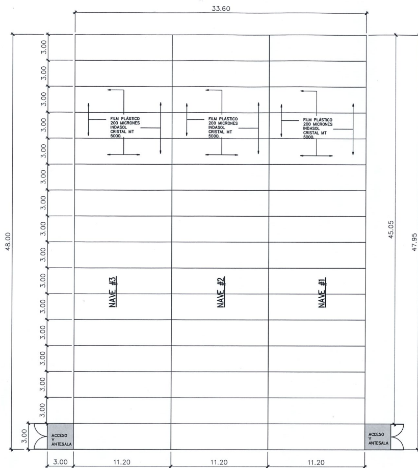
PLANTA ARQ. MODULO I ESC. 1:200
