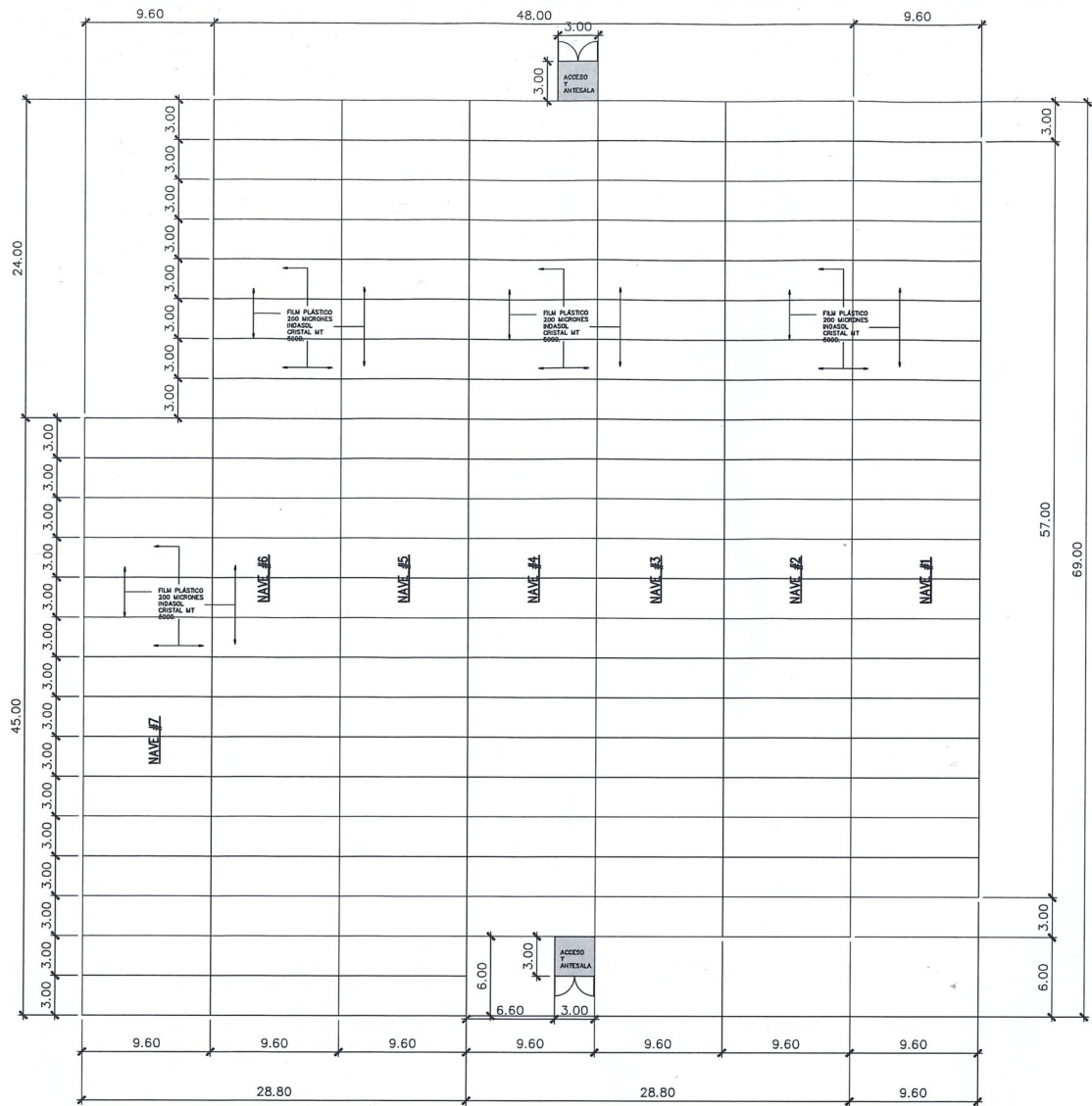
PLANTA ARQ. MODULO II
