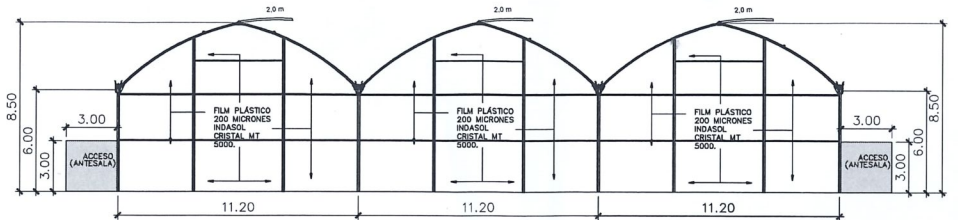
ELEVACION POSTERIOR MODULO I ESC. 1:200
