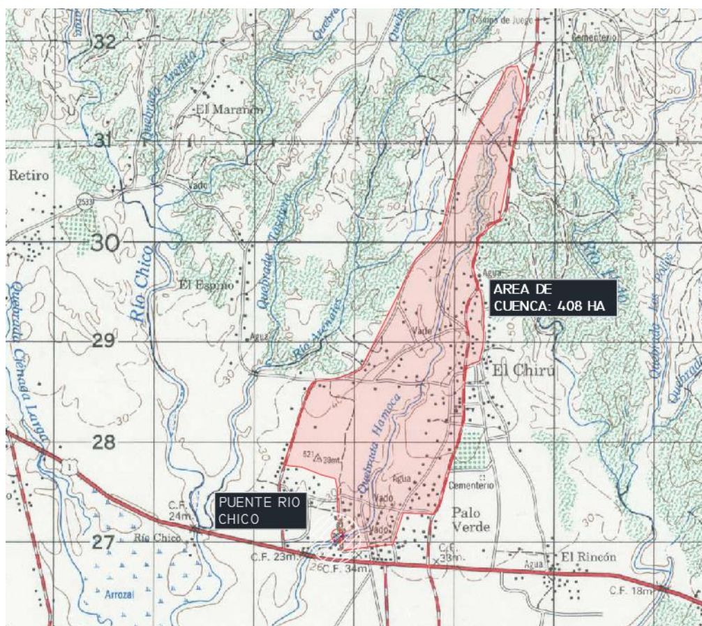
Imagen 2. Delimitación de la Cuenca Base Tomy Guardia
