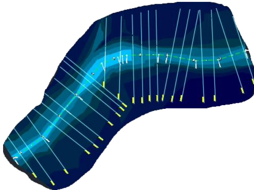
Imagen No. 7. Generación de Surface para construir Secciones Transversales.
