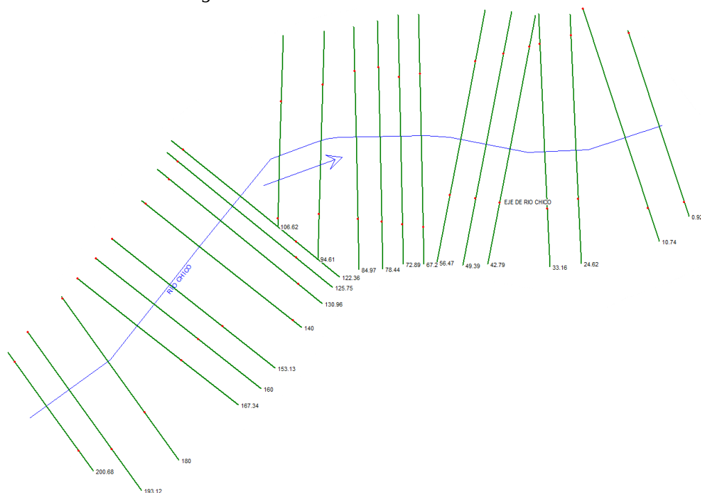
Imagen No. 8. Planta Geométrica modelo hec ras
