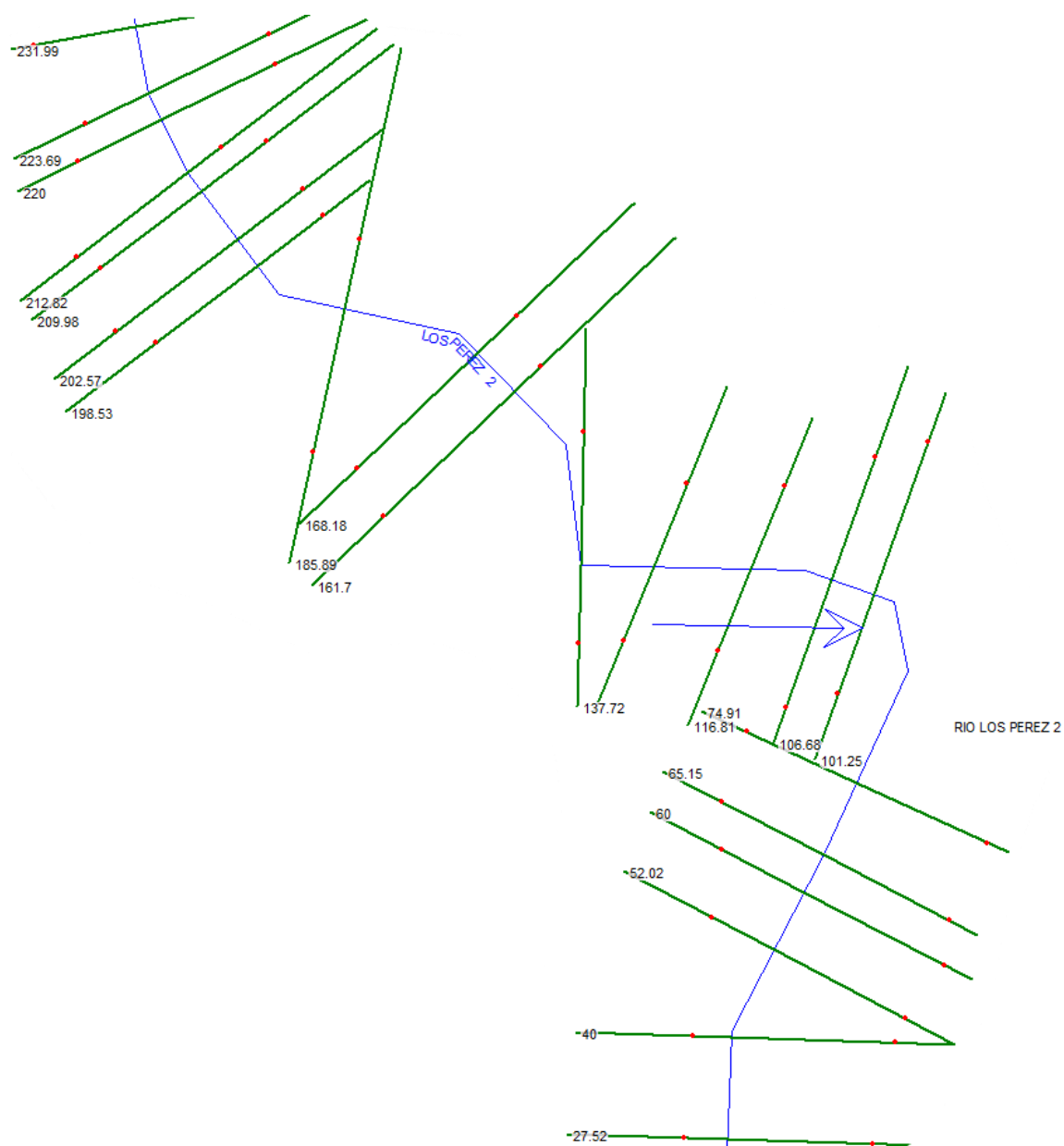
Imagen No. 8. Planta Geométrica modelo hec ras
