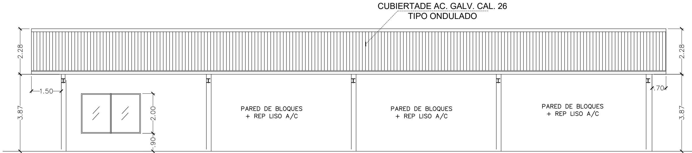
ELEVACION LATERAL DERECHA ESCALA=1:75
