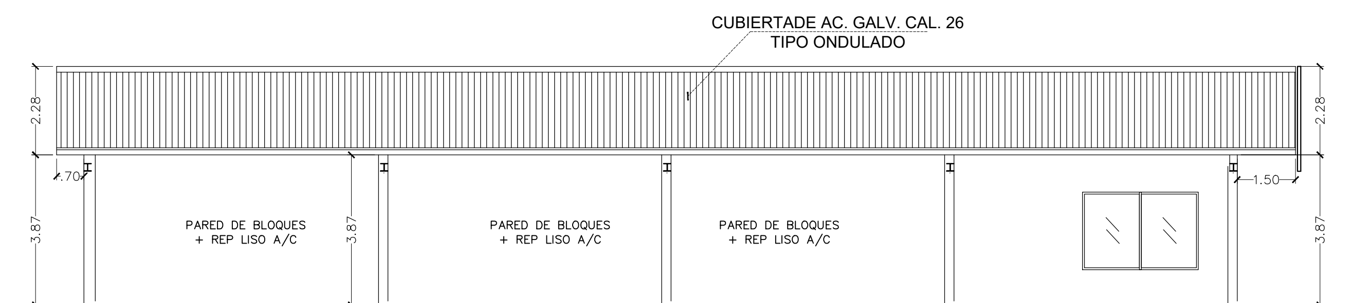
ELEVACION LATERAL IZQUIERDA ESCALA=1:75
