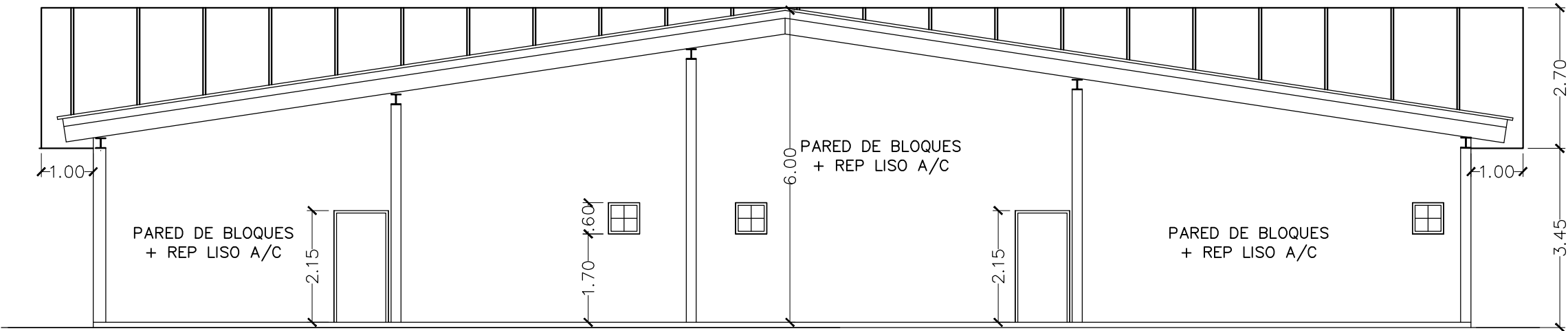
ELEVACION POSTERIOR ESCALA=1:75
