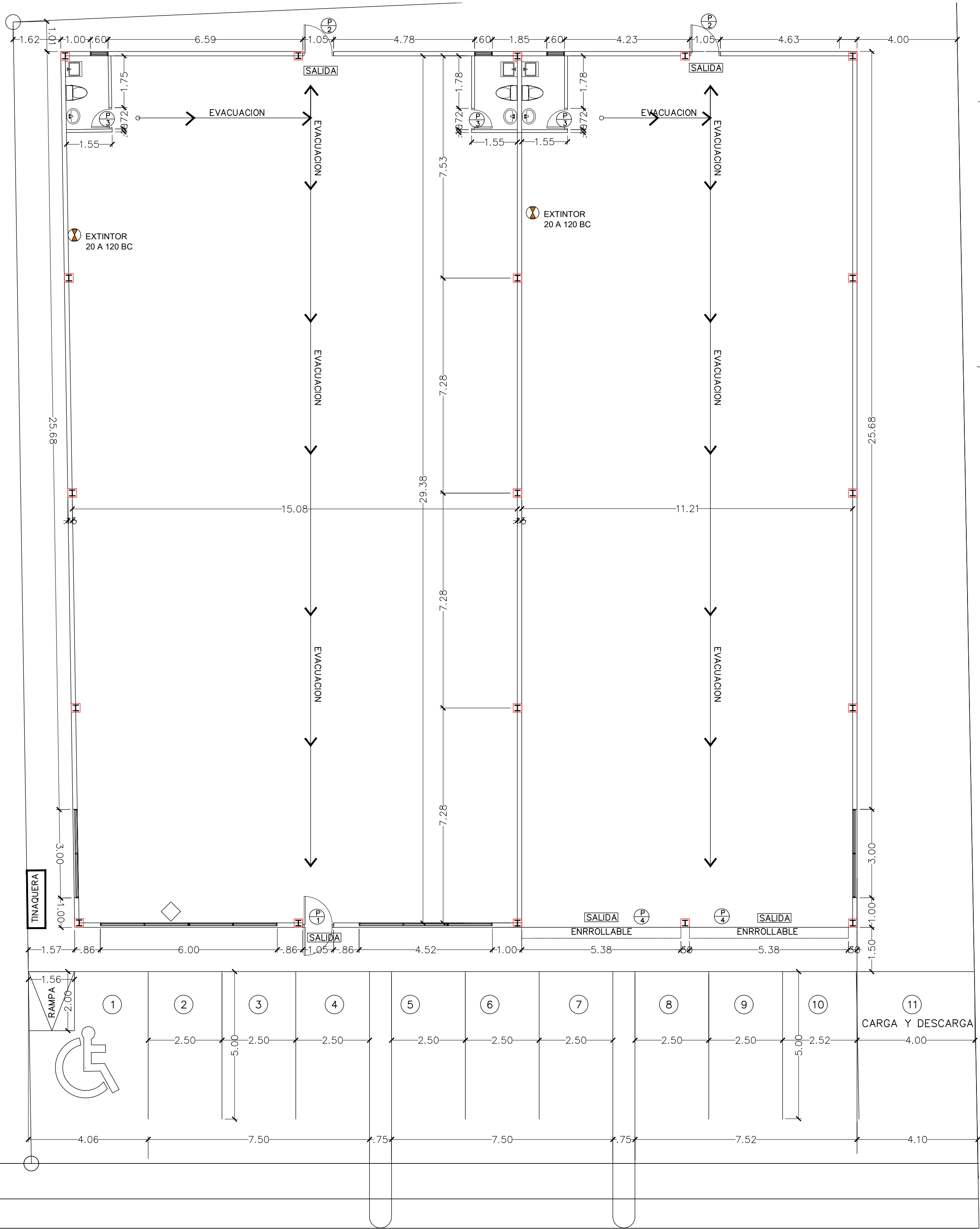
PLANTA ARQUITECTONICA ESCALA=1:100
