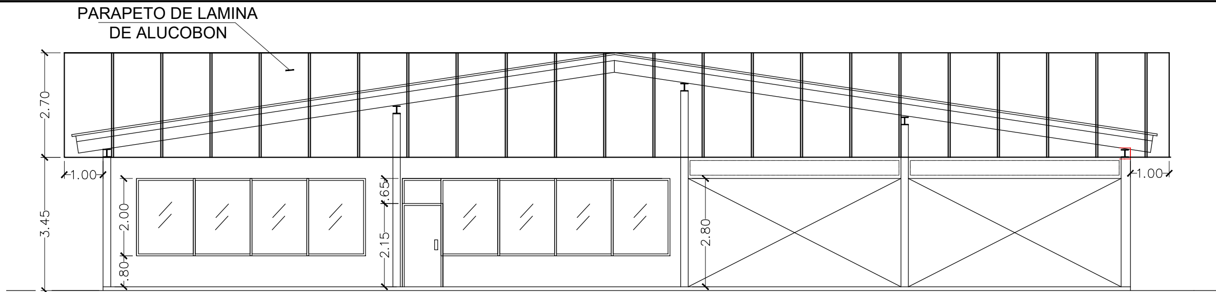
ELEVACION FRONTAL ESCALA=1:75
