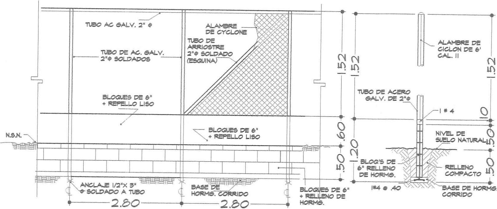
DET. TIPICO DE CERCA DE MALLA CICLON ESCALA 1:40
