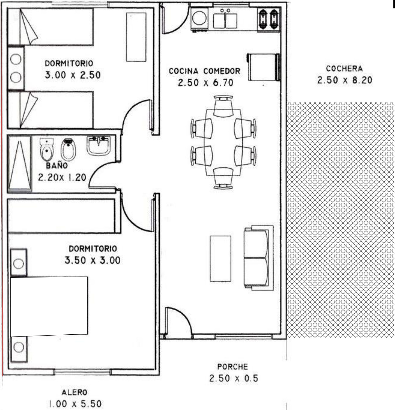
VISTA DE PLANTA
