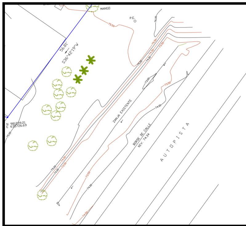
Imagen N°3. Vista de planta del proyecto
