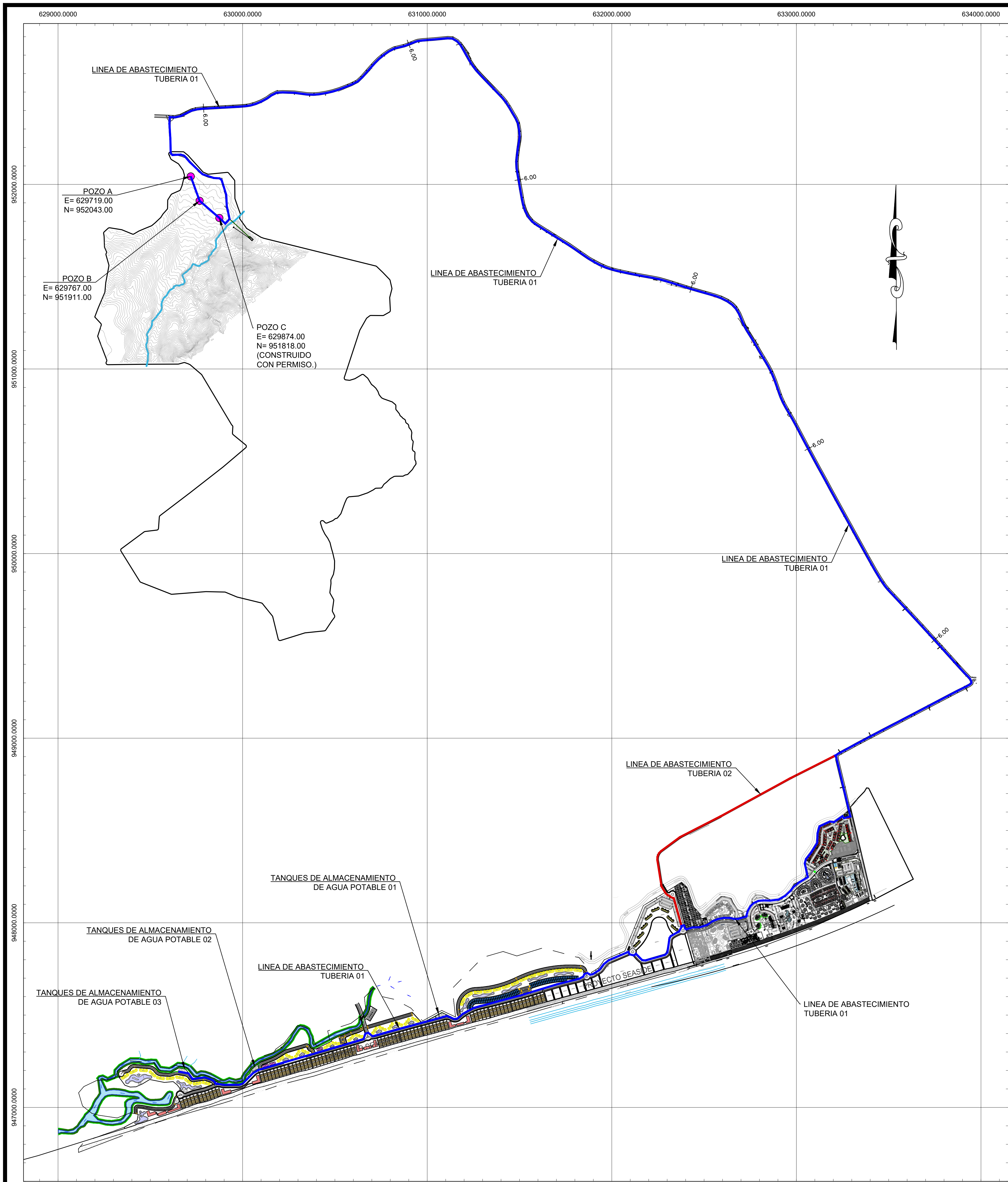
PLANTA GENERAL LOCALIZACION DE LINEA DE ABASTECIMIENTO DE AGUA POTABLE, DESDE PUNTO DE GENERACION (POZOS) HASTA TANQUES DE ALMACENAMIENTO. ESCALA 1: 10,000
