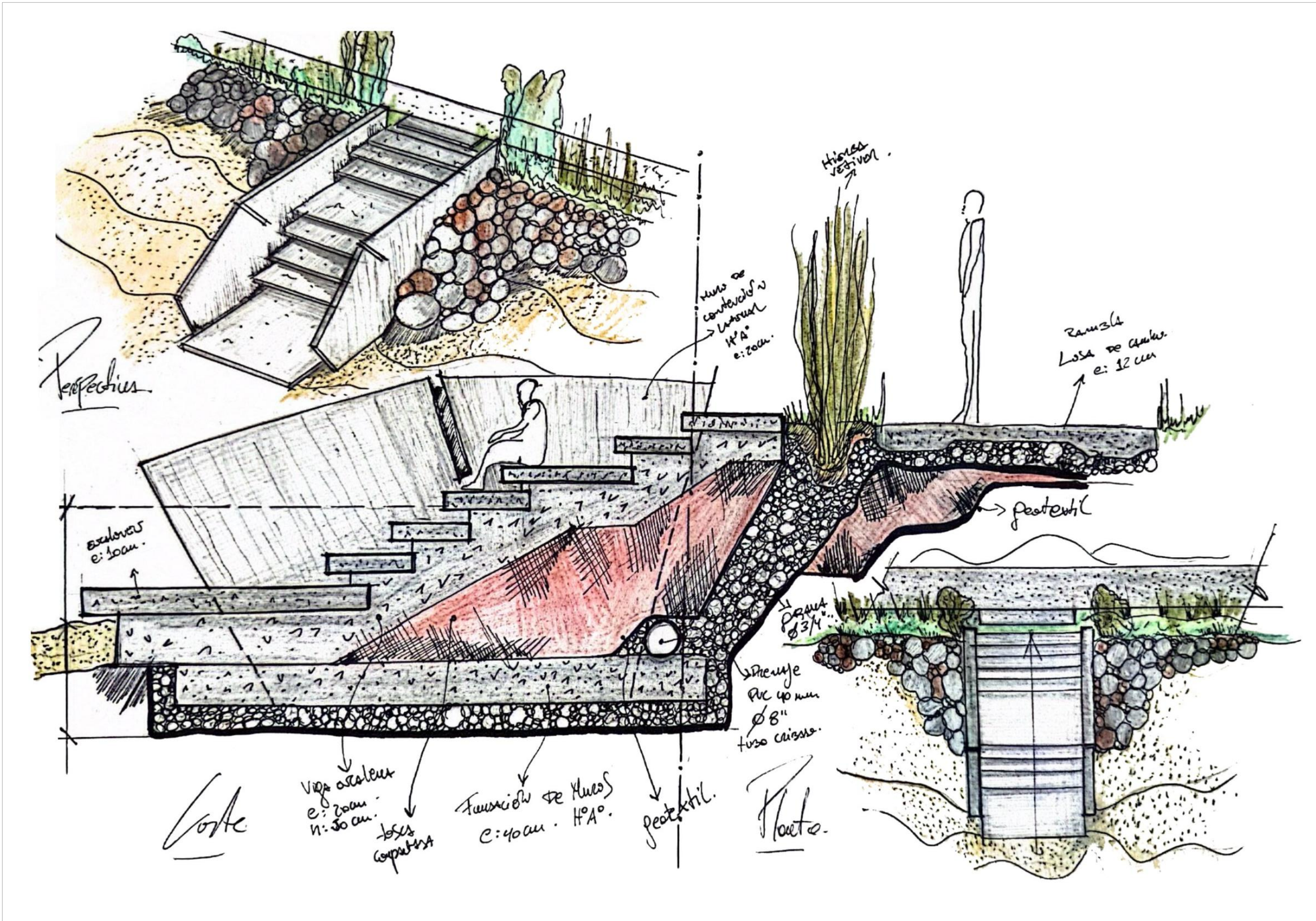
CROQUIS ESCOLLERA TIPO "F"
