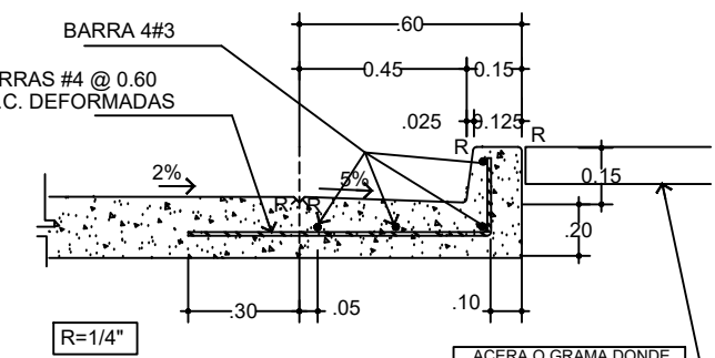
DETALLE DE CORDON/CUNETETA
