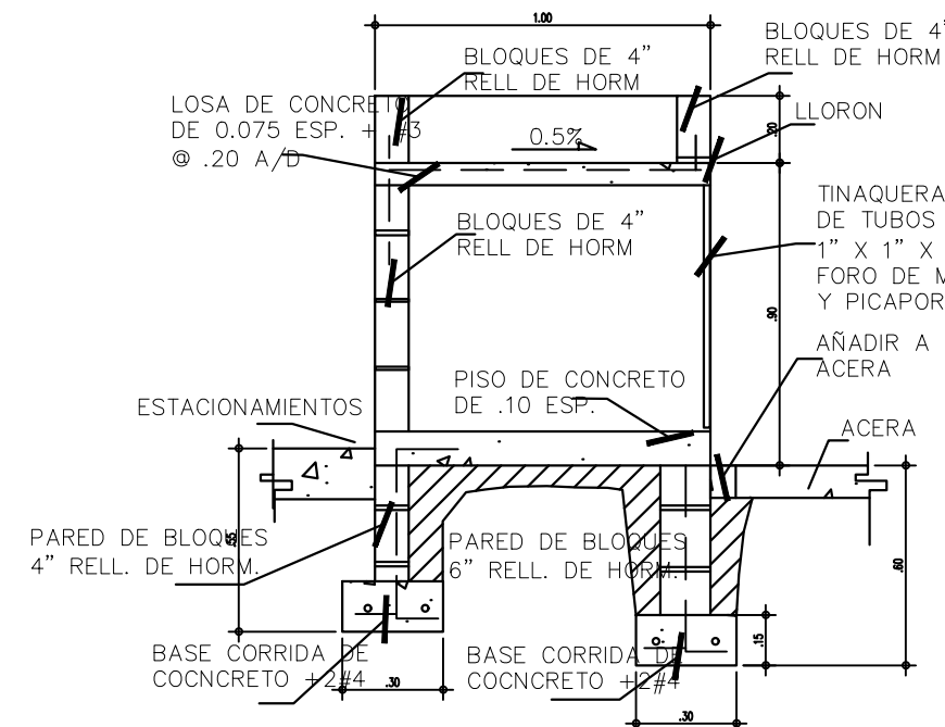
SECCION DE TINAQUERA ESCALA : 1/25
