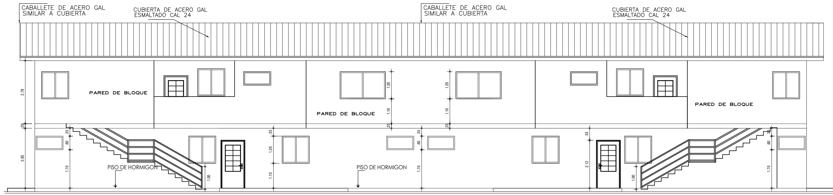
ELEVACIÓN POSTERIOR
