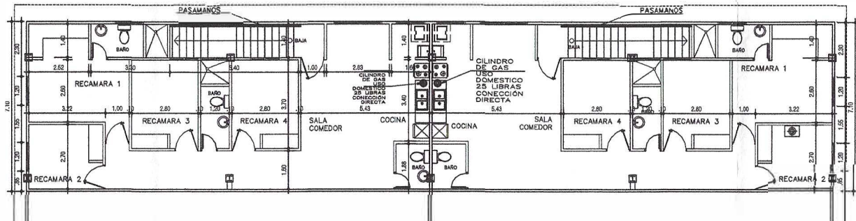
PLANTA ARQUITECTONICA PLANTA ALTA MEZANINE ESC. 1:100
