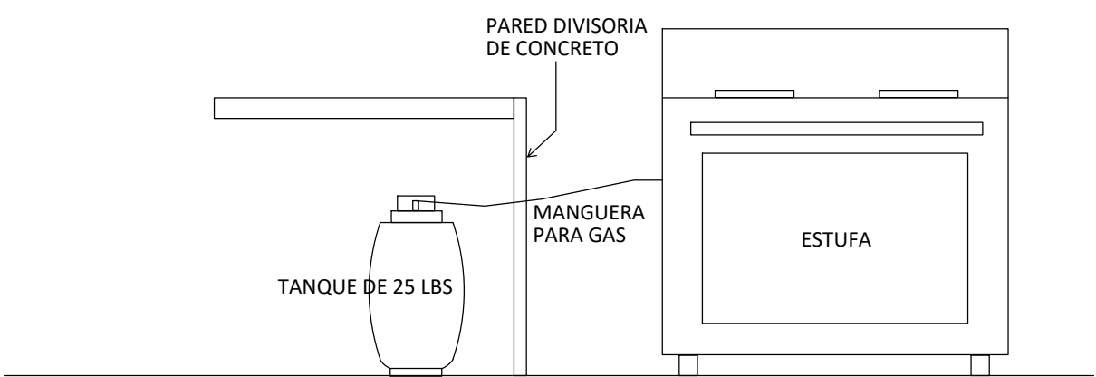
DETALLE DE CONEXION DE DE TANQUE DE GAS DE 25 LBS A ESTUFA
