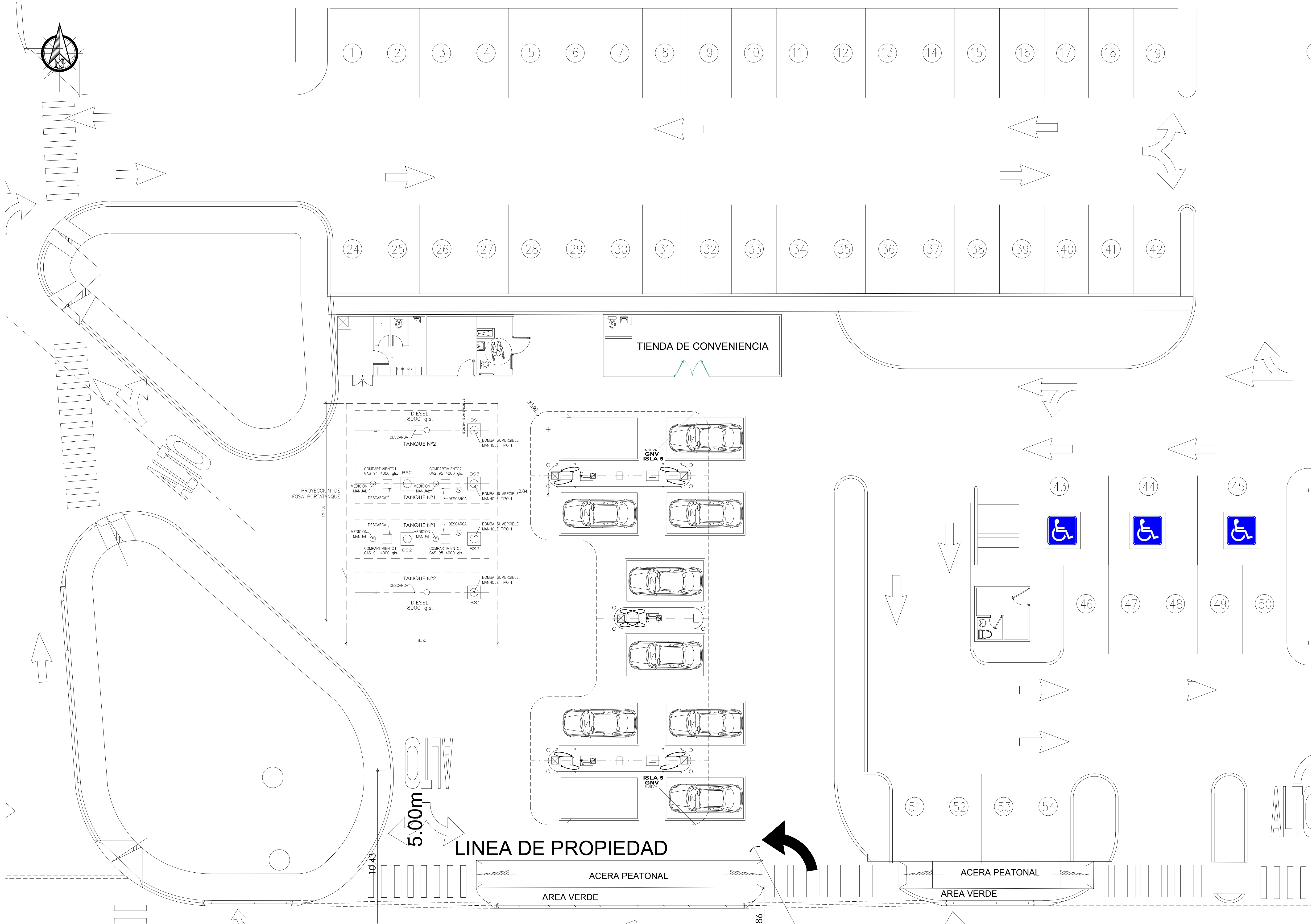
PLANTA ARQUITECTONICA ESTACION DE COMBUSTIBLE
