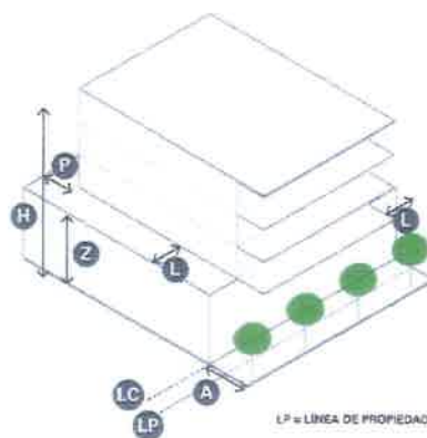
DIAGRAMA ESQUEMÁTICO
