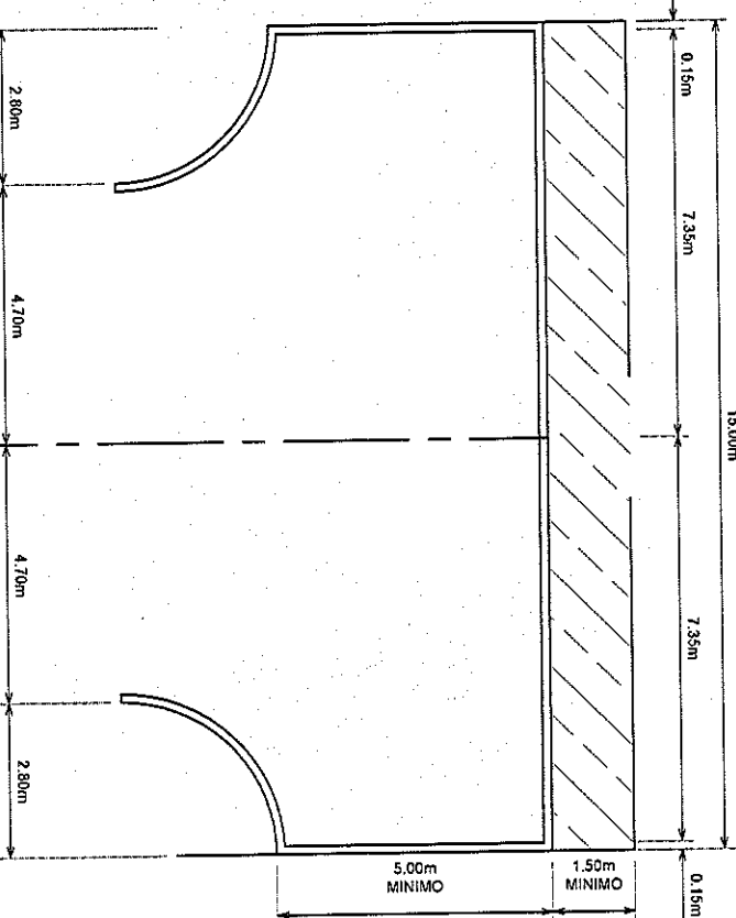
DETALLE DE MARTILLO CALLE DE 12.80 mts.
