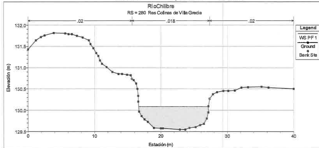
Vista 13: Estación 280.00 – Quebrada Sin Nombre
