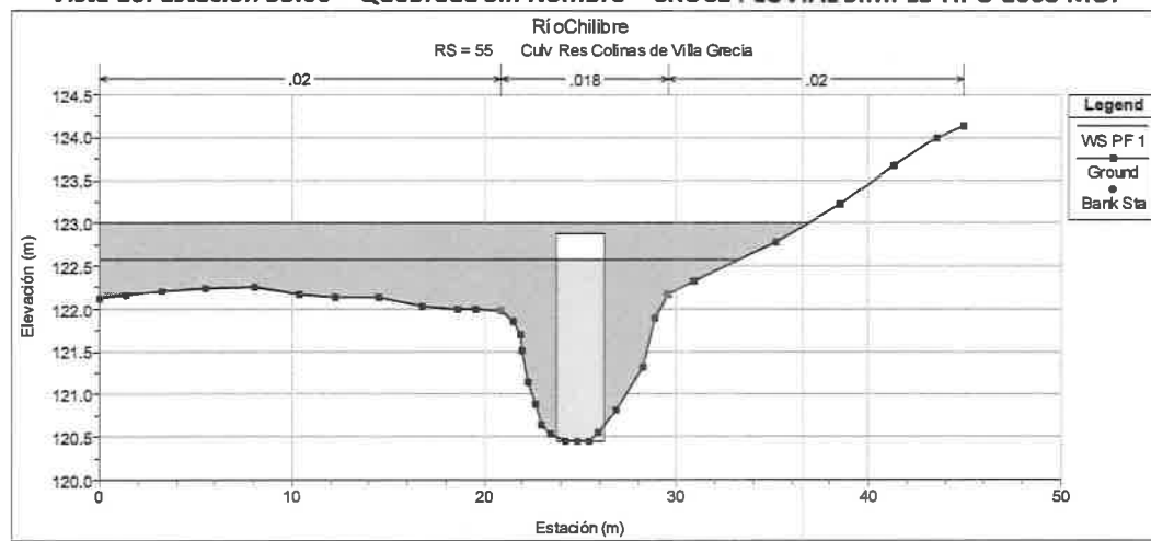
Vista 16: Estación 55.00 – Quebrada Sin Nombre – CRUCE PLUVIAL SIMPLE TIPO 1008 MOP
