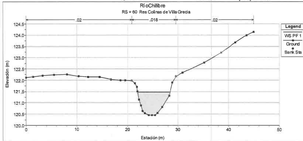
Vista 15: Estación 60.00 – Quebrada Sin Nombre – Cruce Pluvial propuesto
