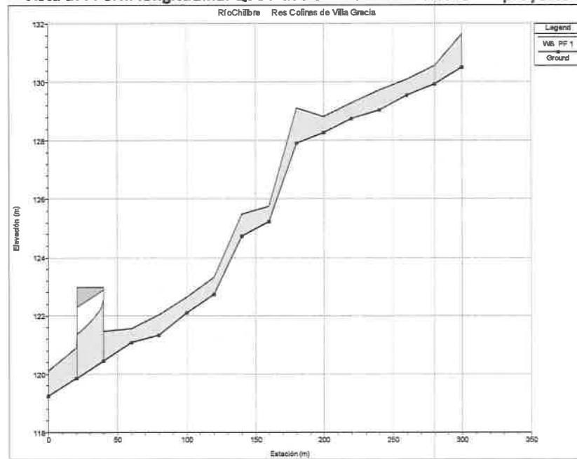
Vista 18: Perfil longitudinal Quebrada Río Chilbre – Tramo del Proyecto
