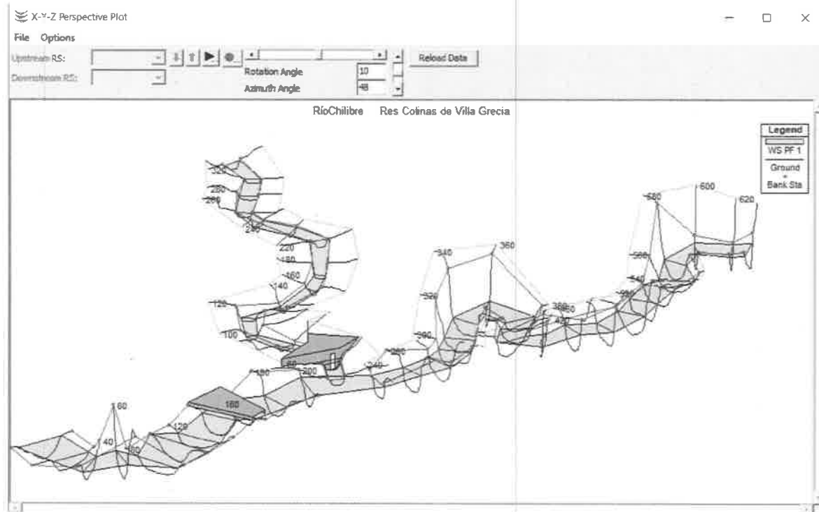
Vista 2: Modelo 2D de las fuentes analizadas vs niveles de inundación.
