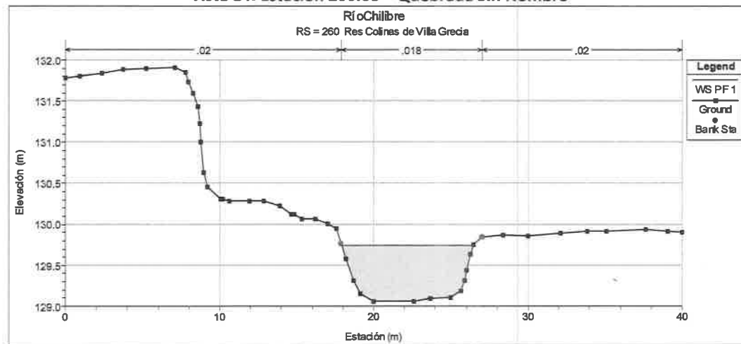
Vista 14: Estación 260.00 – Quebrada Sin Nombre
