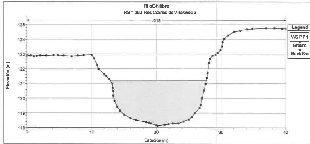
Vista 11: Estación 260.00 – Río Chilibre
