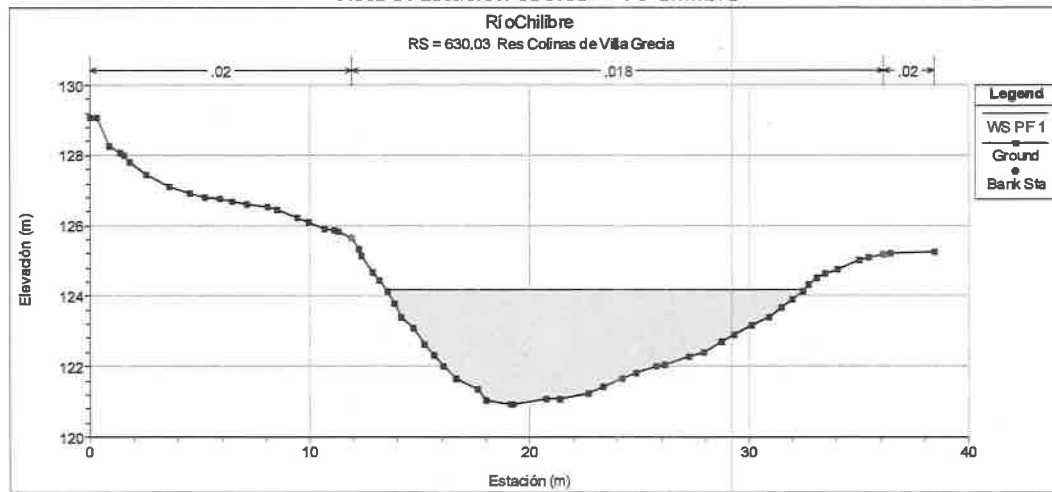
Vista 9: Estación 630.03 – Río Chilíbre
