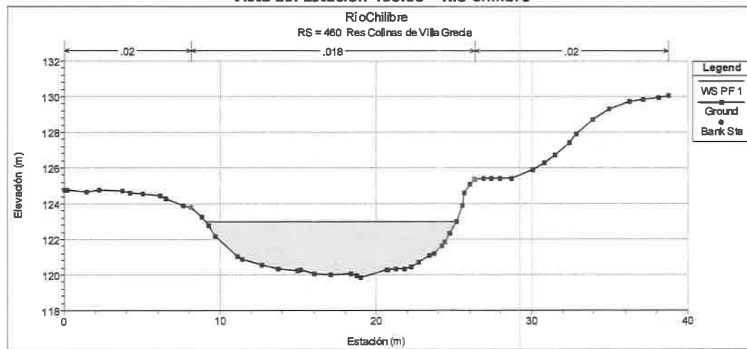
Vista 10: Estación 460.00 – Río Chilíbre
