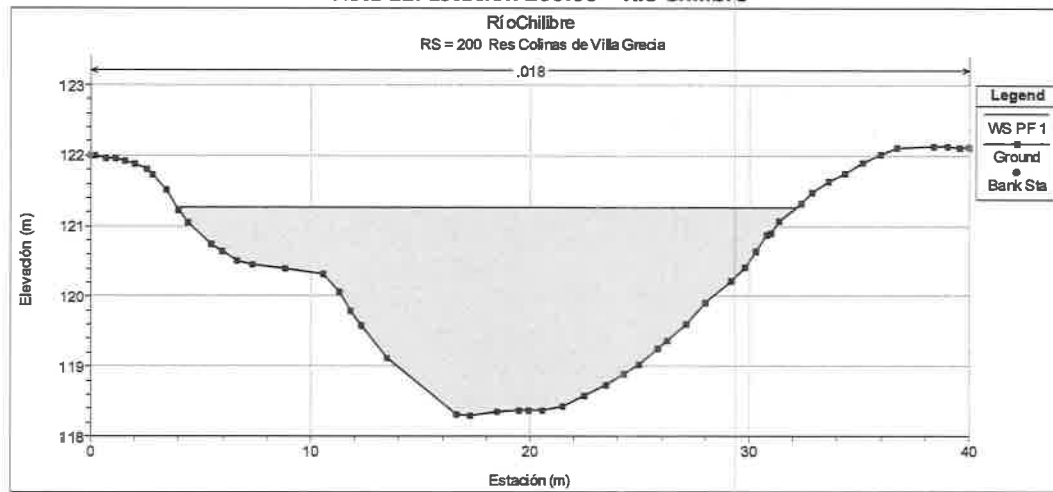
Vista 12: Estación 200.00 – Río Chilibre
