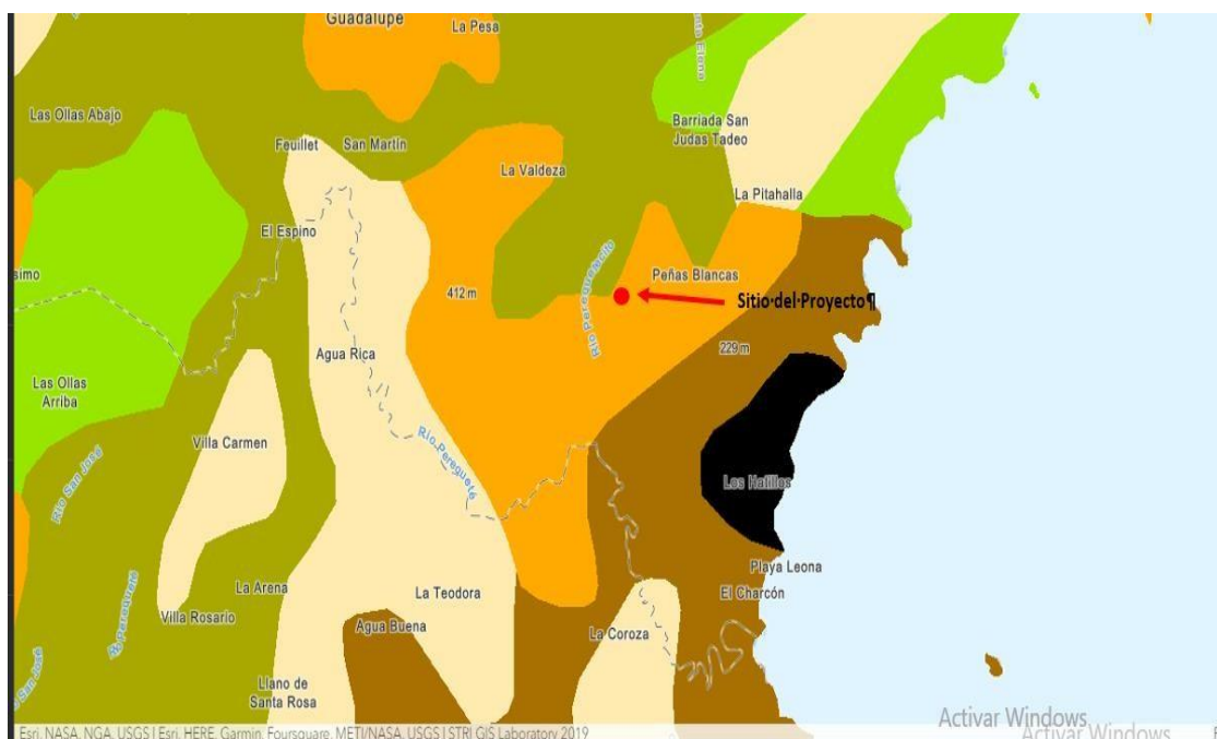
Figura 6.1. Mapa de capacidad agrologica de los suelos.
