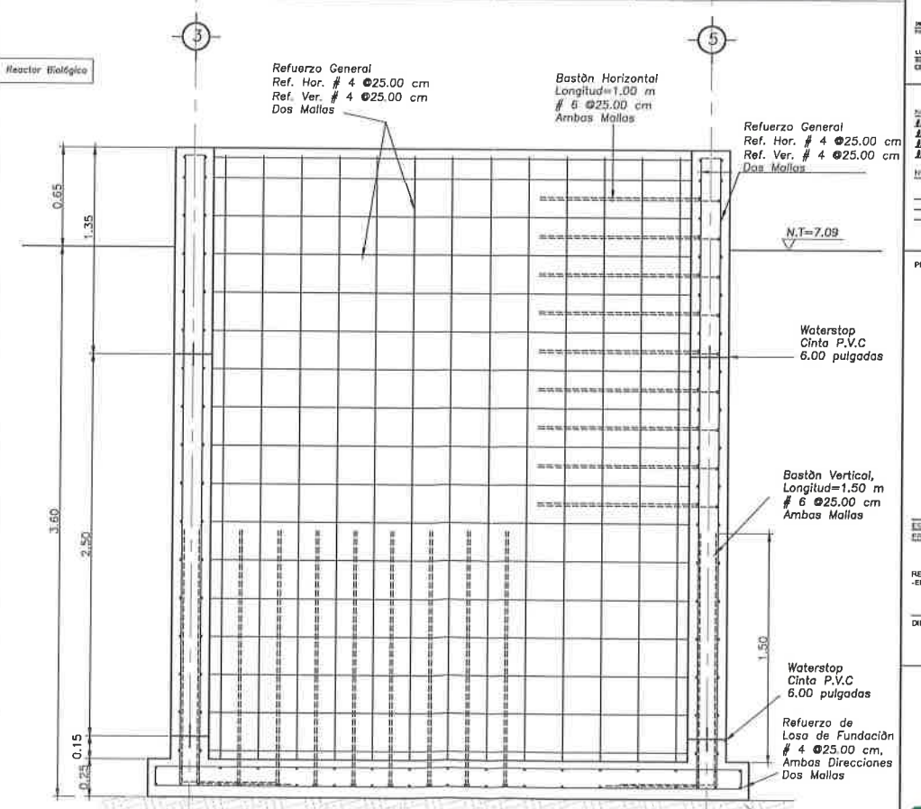
ELEVACION ESTRUCTURAL EJE-C
