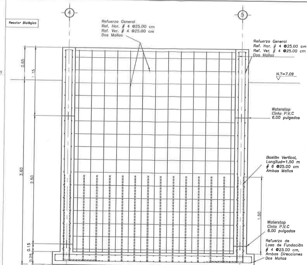
ELEVACION ESTRUCTURAL EJES-G
