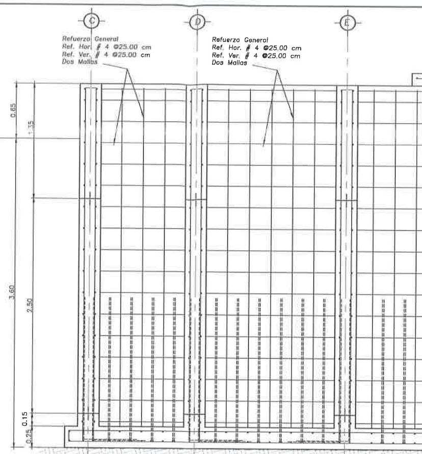
ELEVACION ESTRUCTURAL EJE-4
