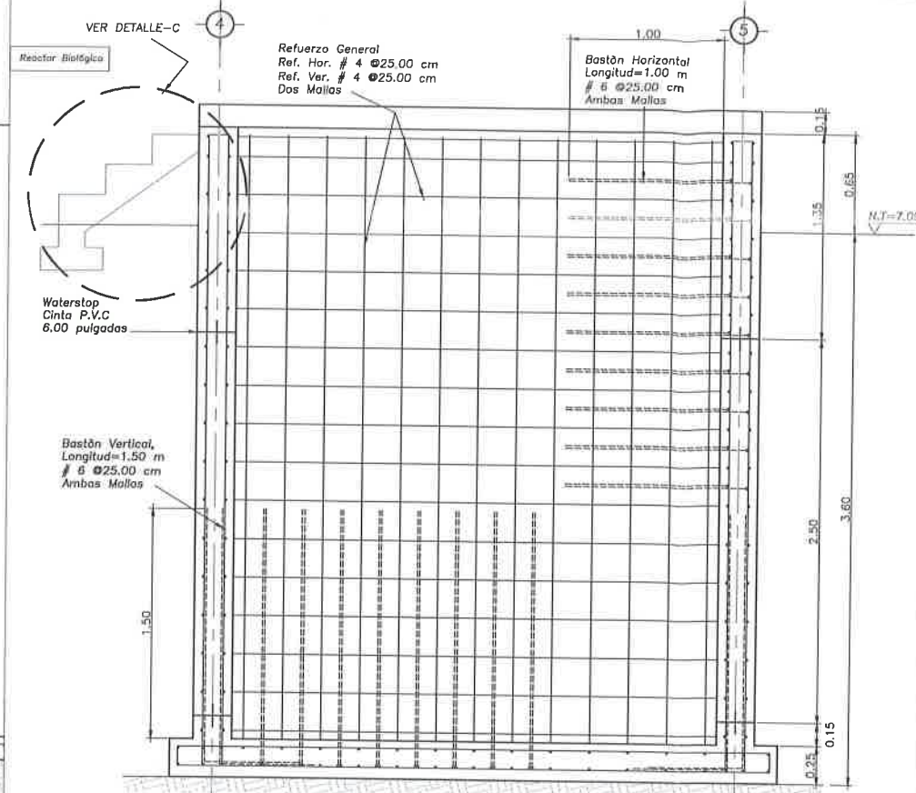
ELEVACION ESTRUCTURAL EJES-F
