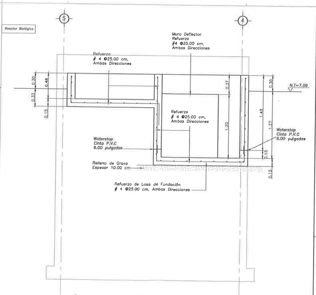
SECCION ESTRUCTURAL G-G
