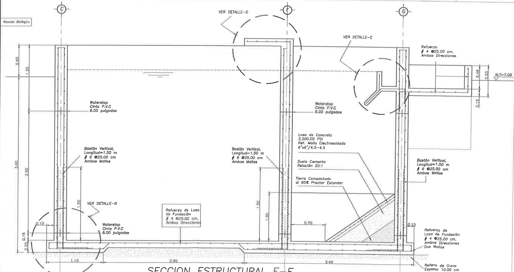
SECCION ESTRUCTURAL F-F
