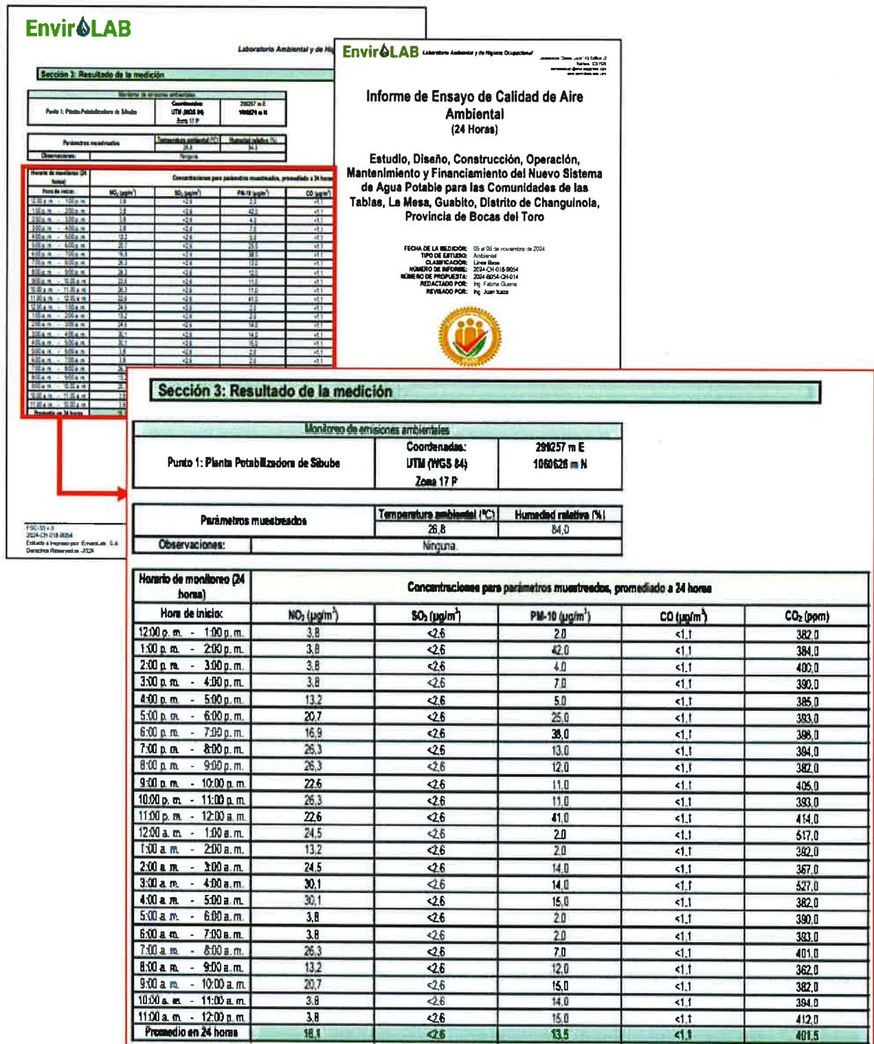
Figura 23. Resultados Monitoreo Calidad de Aire 24 horas - Comunidad de Sibube.
