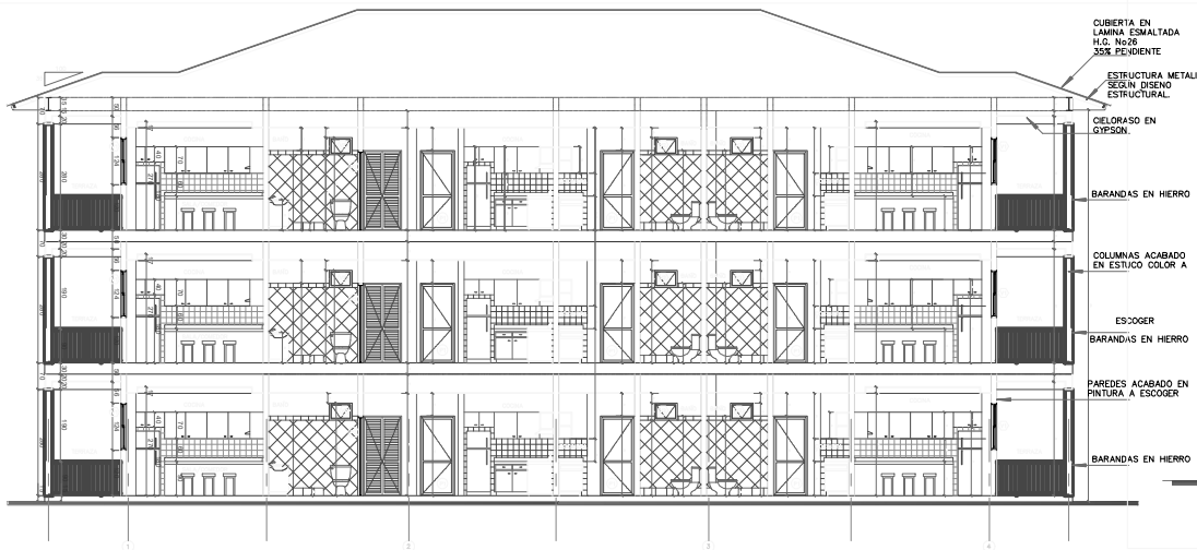
SECCION LONGITUDINAL ESC:1/100
