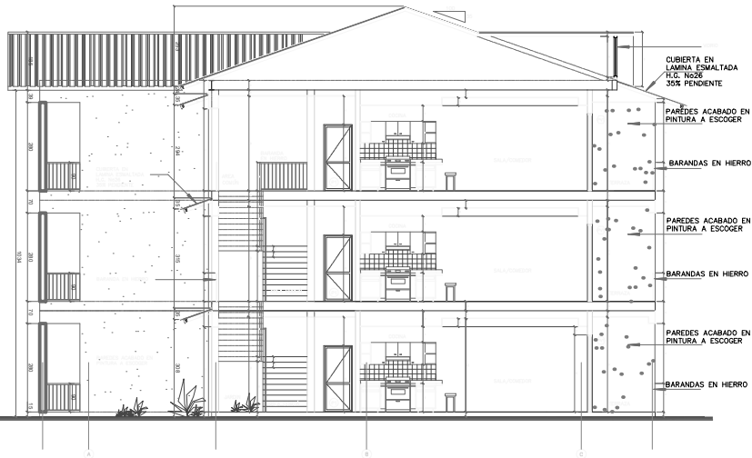
SECCION TRANSVERSAL ESC:1/100
