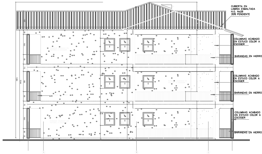
ELEVACION LATERAL IZQUIERDA ESC:1/100
