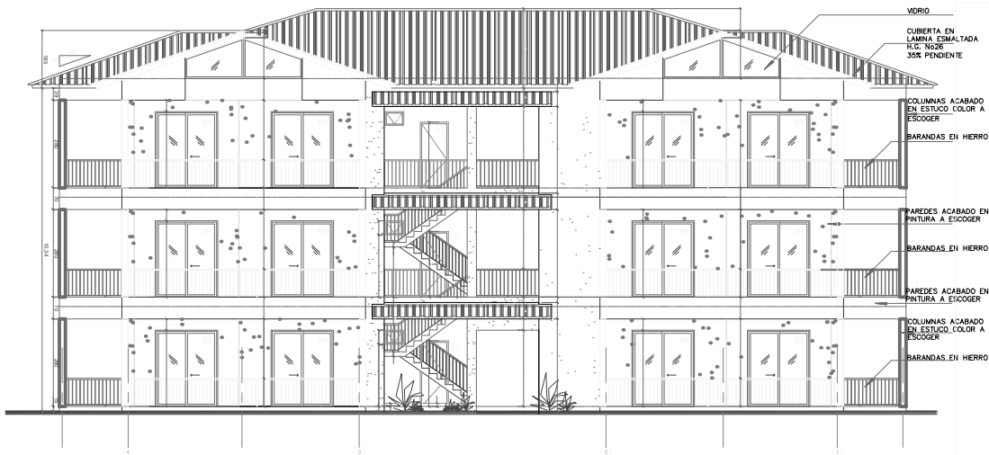
ELEVACION FRONTAL ESC:1/100
