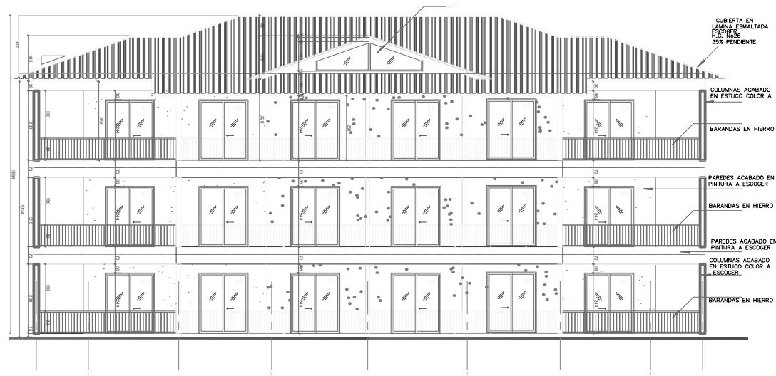
ELEVACION POSTERIOR ESC:1/100
