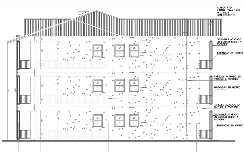
ELEVACION LATERAL DERECHA ESC:1/100
