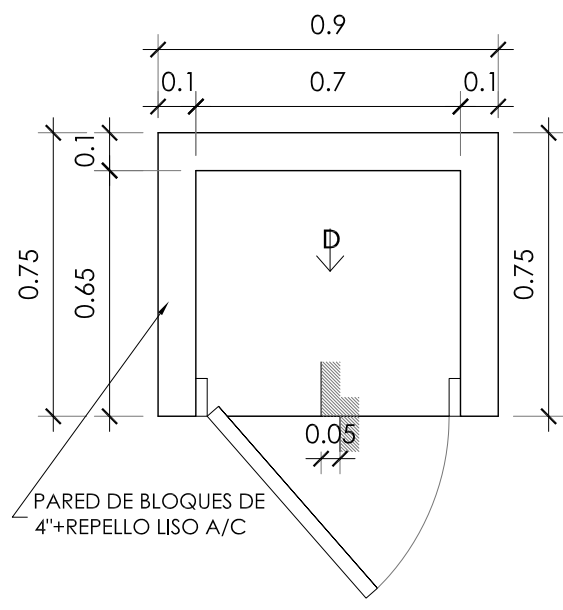
PLANTA BASURERO ESCALA: 1:20
