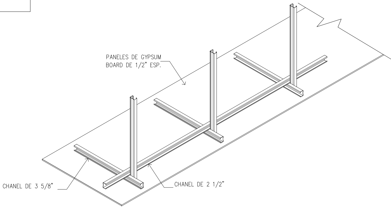
ISOMETRICO DE CIELO RASO DE GYPSUM BOARD C
