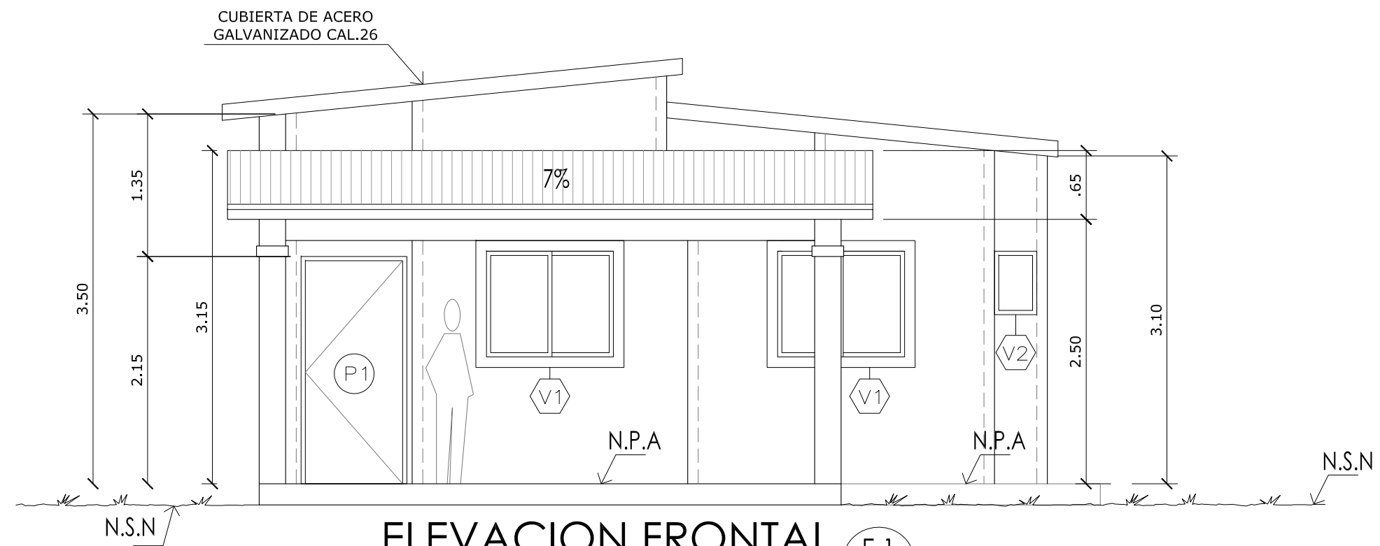
ELEVACION FRONTAL E-1 A003 ESCALA 1:50
