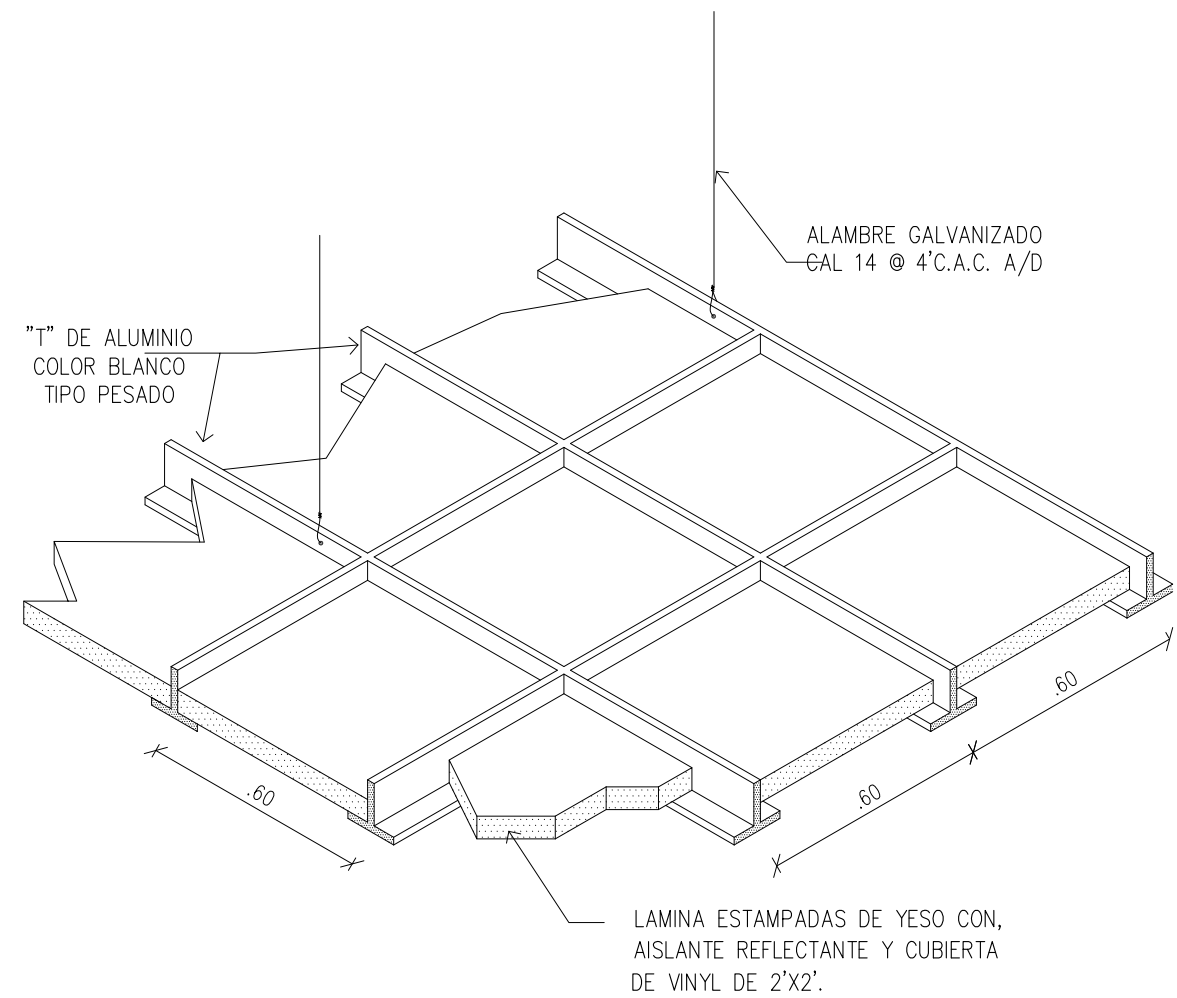
ISOMETRICO DE CIELO RASO DE LAMINA ESTAMPADA S/E
