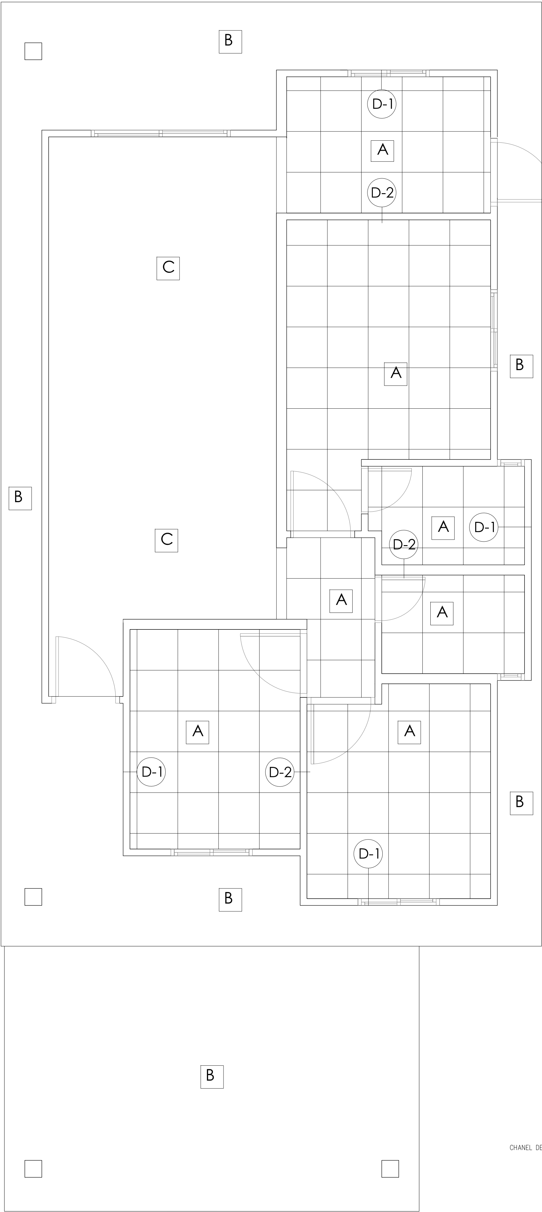
PLANTA DE CIELO RASO VIVIENDAS LOTES 9 Y 10 ESCALA 1:33 1/3
