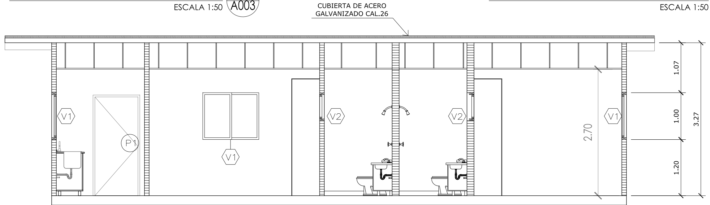
SECCION LONGITUDINAL S-1 A003 ESCALA 1:50
