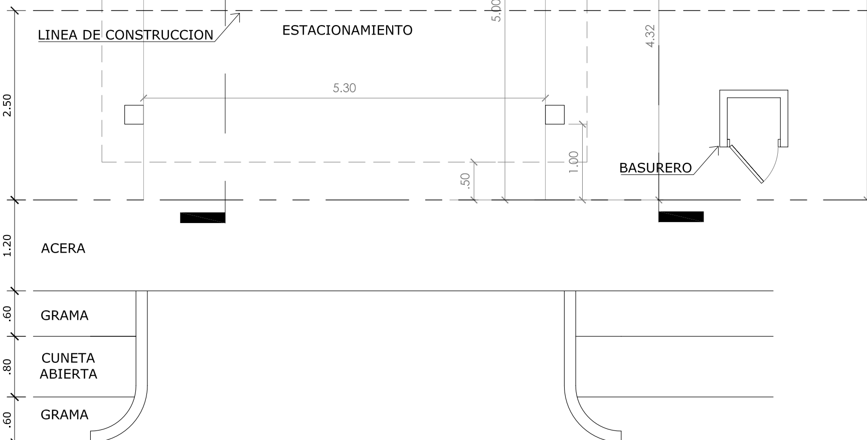
NIVEL 000 VIVIENDAS LOTES 5, 6 Y 7 ESCALA 1:50
