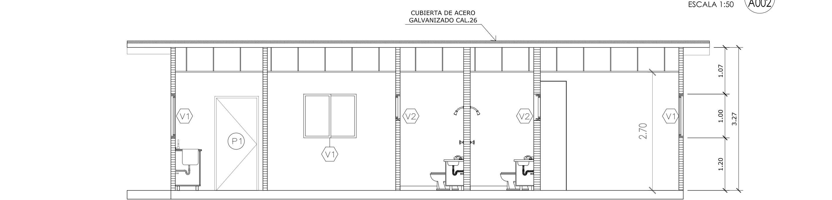
SECCION LONGITUDINAL S-1 A002 ESCALA 1:50
