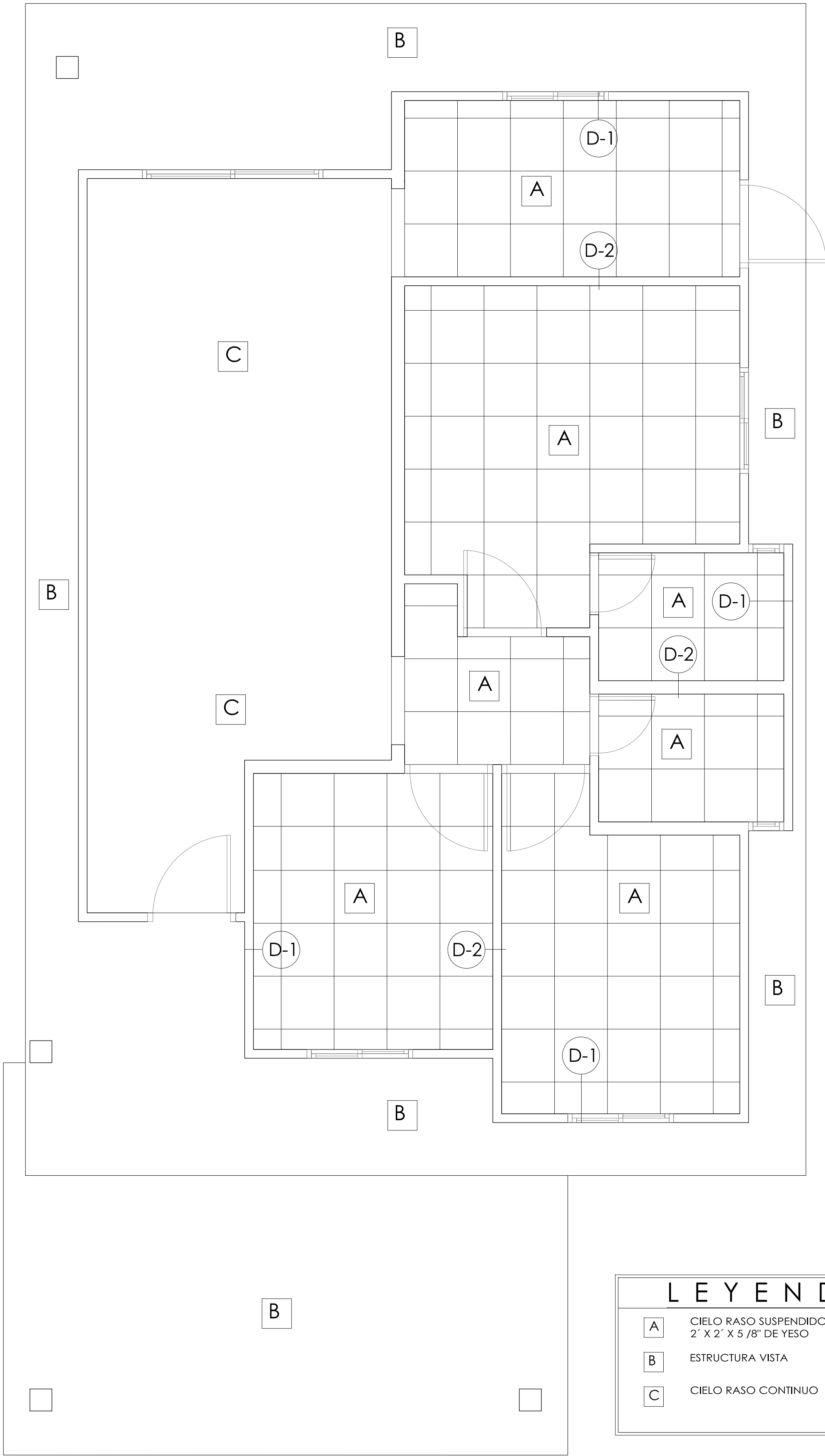
PLANTA DE CIELO RASO VIVIENDAS LOTES 5, 6 Y 7 ESCALA 1:33 1/3
