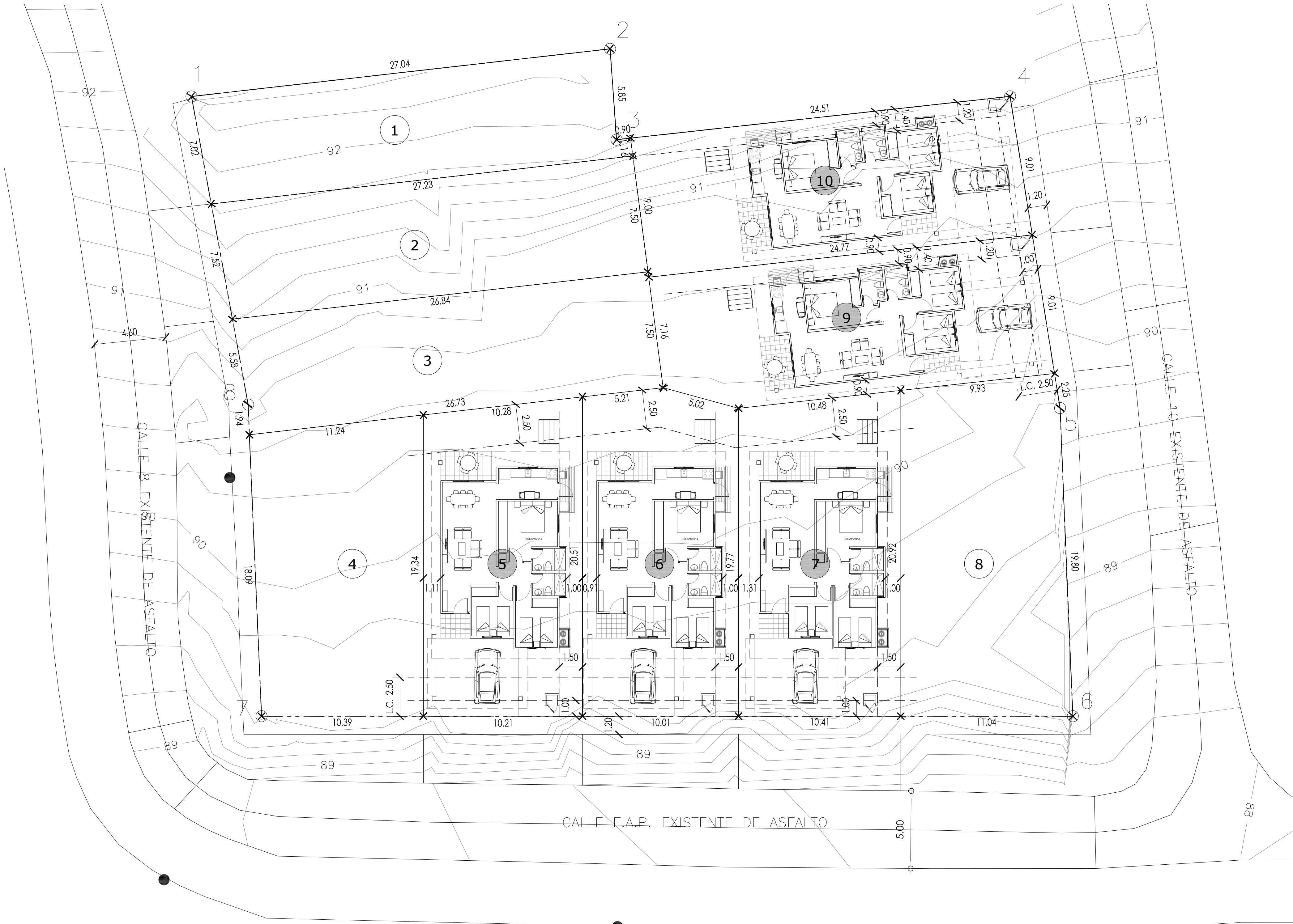
UBICACION EN LOTE ESCALA: 1:150
