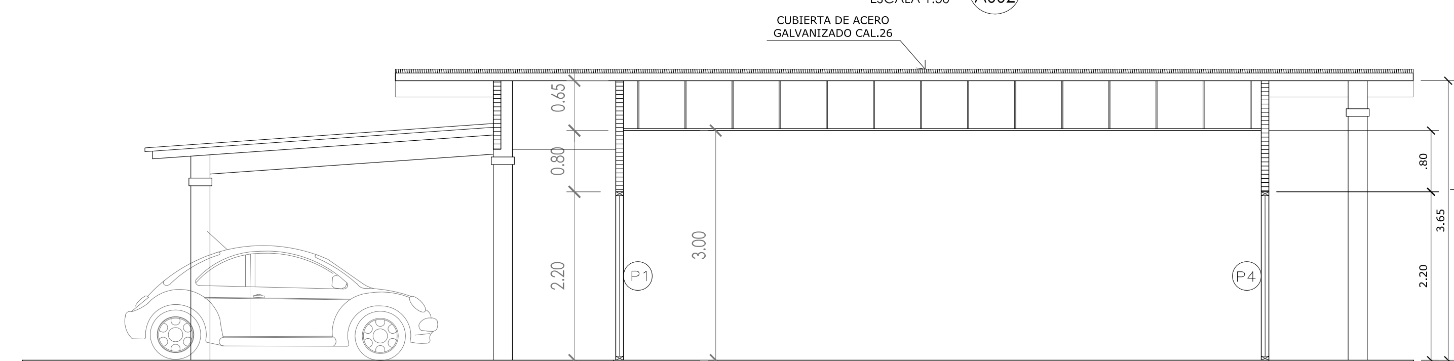
SECCION LONGITUDINAL S-3 A002 ESCALA 1:50
