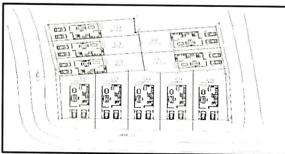
Figura 1. Diez (10) viviendas de dos (2) niveles según el EsIA aprobado
