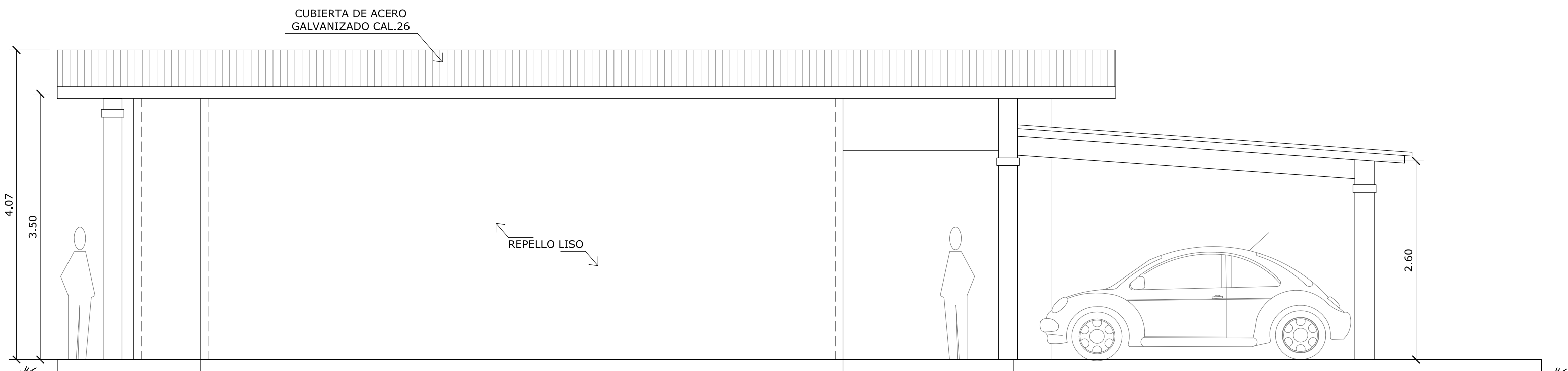
ELEVACION LATERAL IZQUIERDA E-4 A003 ESCALA 1:50
