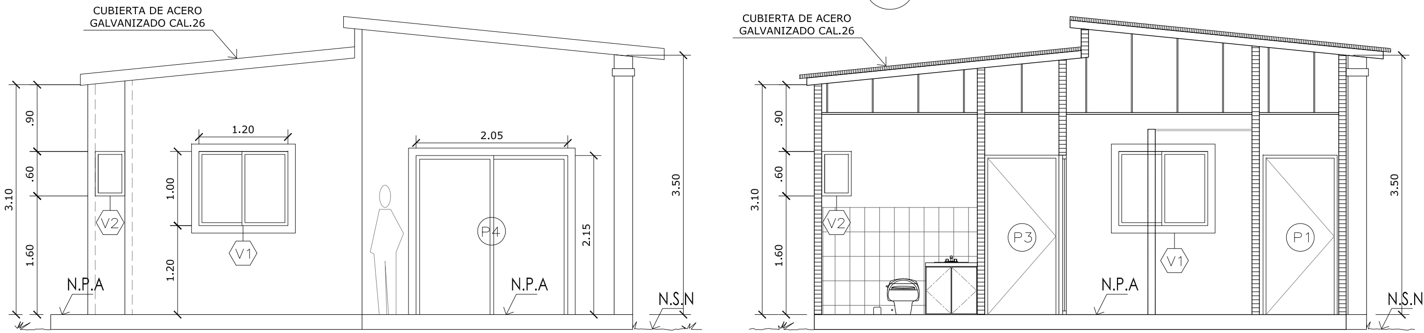
ELEVACION POSTERIOR E-3 A003 ESCALA 1:50
