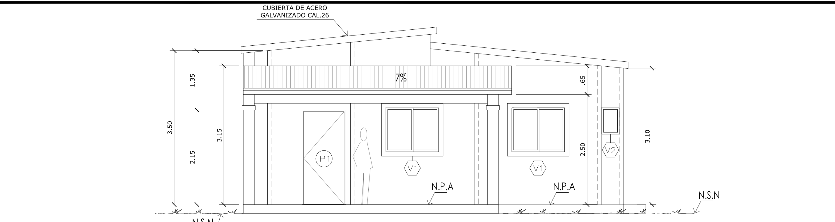
ELEVACION FRONTAL E-1 A002 ESCALA 1:50
