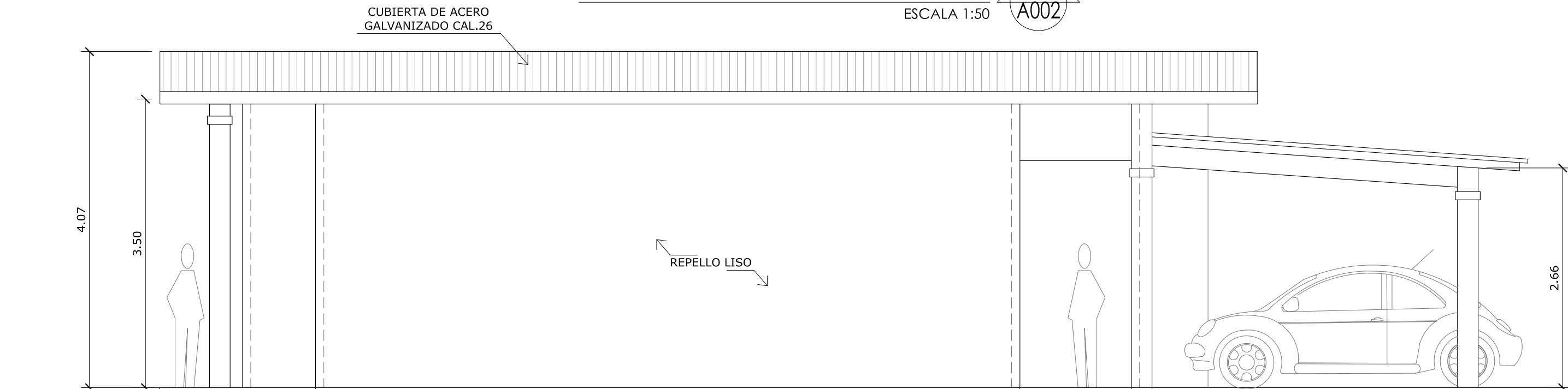
ELEVACION LATERAL IZQUIERDA E-4 A002 ESCALA 1:50
