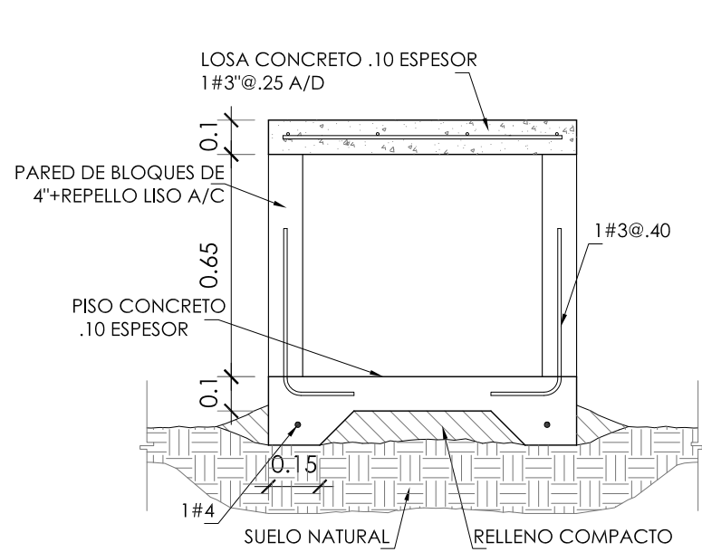
SECCION BASURERO ESCALA: 1:20
