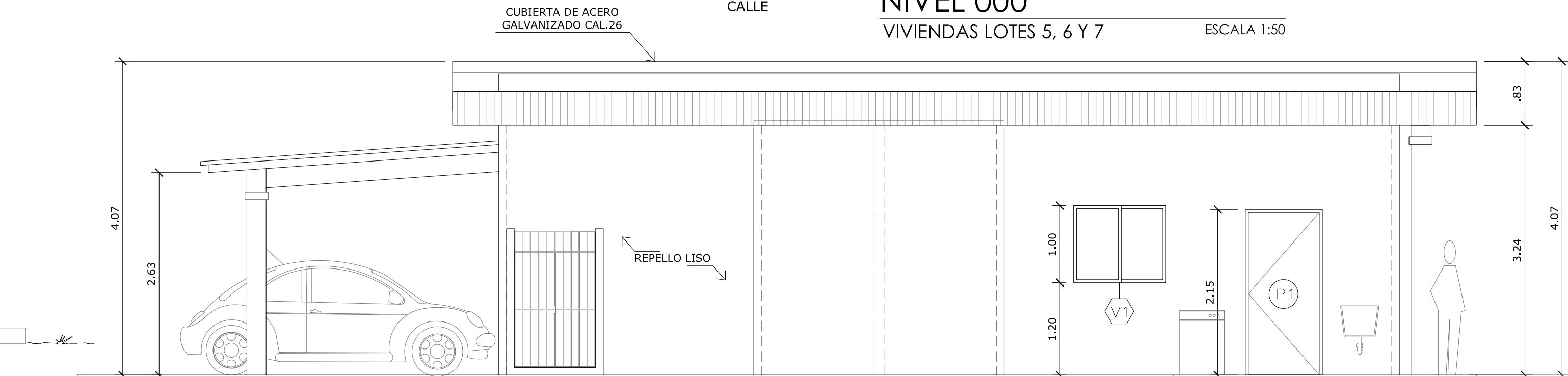
ELEVACION LATERAL DERECHA E-2 A002 ESCALA 1:50
