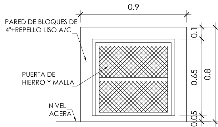
ELEVACION FRONTAL BASURERO ESCALA: 1:20
