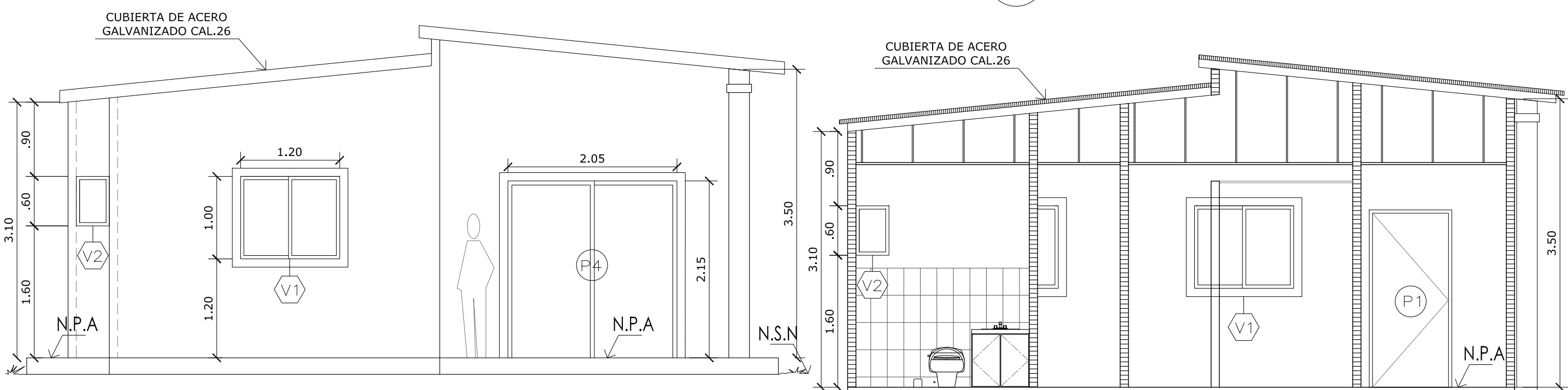
ELEVACION POSTERIOR E-3 A002 ESCALA 1:50
