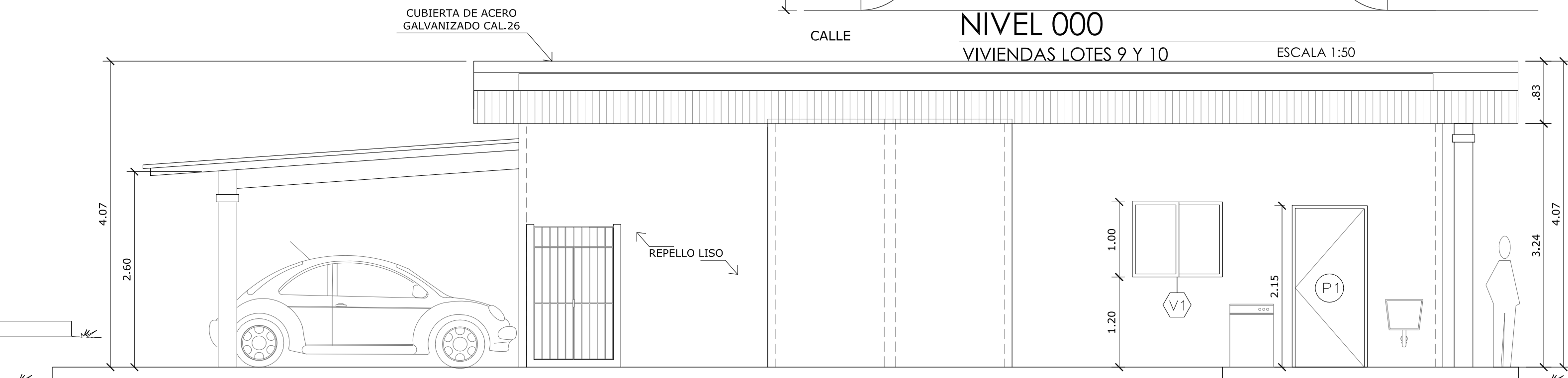
ELEVACION LATERAL DERECHA E-2 A003 ESCALA 1:50
