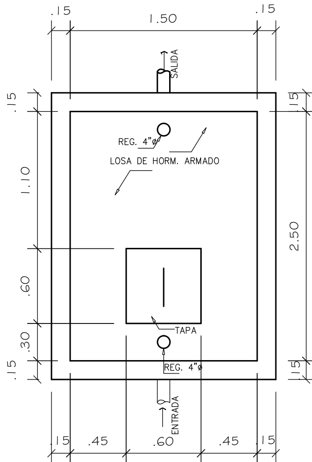
PLANTA DE TANQUE ESCÉPTICO
