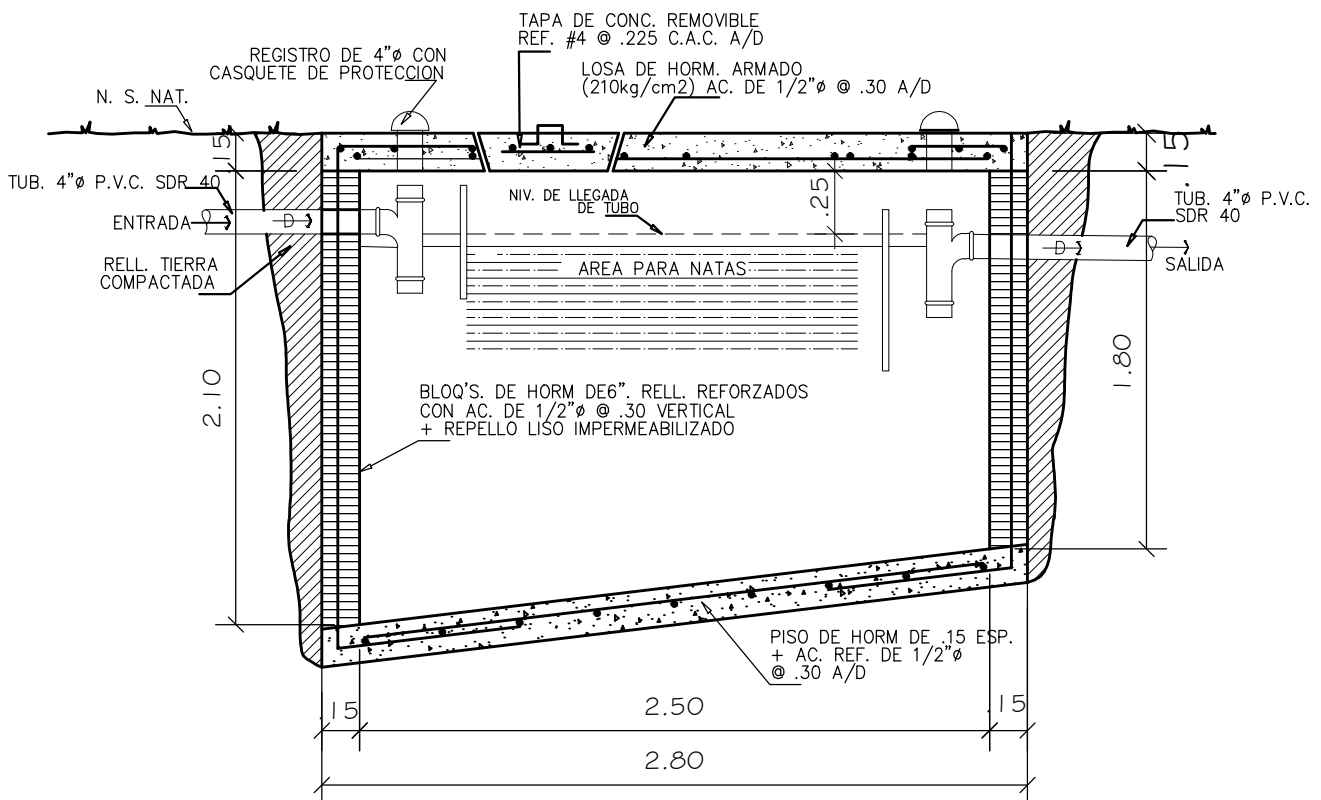
SECCIÓN DE TANQUE ESCÉPTICO
